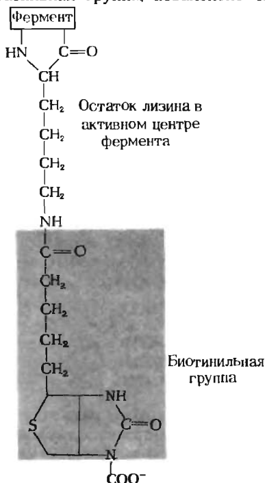
Рис. 16-17. Простетическая группа пируваткарбоксилазы. Карбоксильная группа биотина образует пептидную связь с \epsilon -аминогруппой остатка лизина, входящего в состав активного центра фермента. \text{CO}_2 активируется, образуя N-карбоксипроизводное биотинильной простетической группы. Затем эта карбоксильная группа непосредственный донор \text{CO}_2 для пирувата – переносится на пируват.
