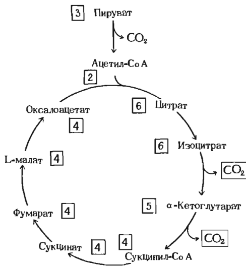
Рис. 16-6. Схема цикла лимонной кислоты. В красных рамках указано число атомов углерода в соответствующих промежуточных продуктах. Четыре атома углерода сукцинил-СоА содержатся в сукцинильной группе, т.е. в той части молекулы, из которой образуется свободный сукцинат.
