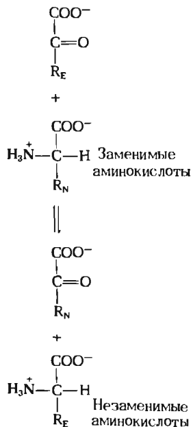
Рис. 19–24. Аминирование \alpha -кетоналогов незаменимых аминокислот (индекс E) в реакциях трансаминирования с заменимыми аминокислотами (индекс N).
