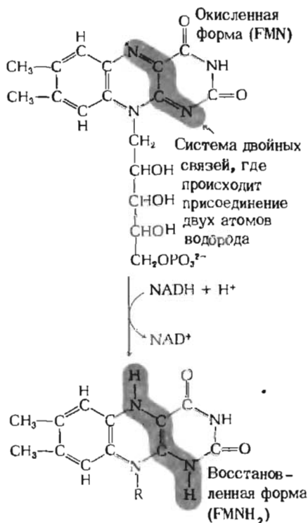
Рис. 17-8. Перенос восстановительных эквивалентов от NADH на флавиноннуклеотид (FMN) — простетическую группу NADH-дегидрогеназы. R означает здесь пятиуглеродную фосфорилированную боковую цепь.
