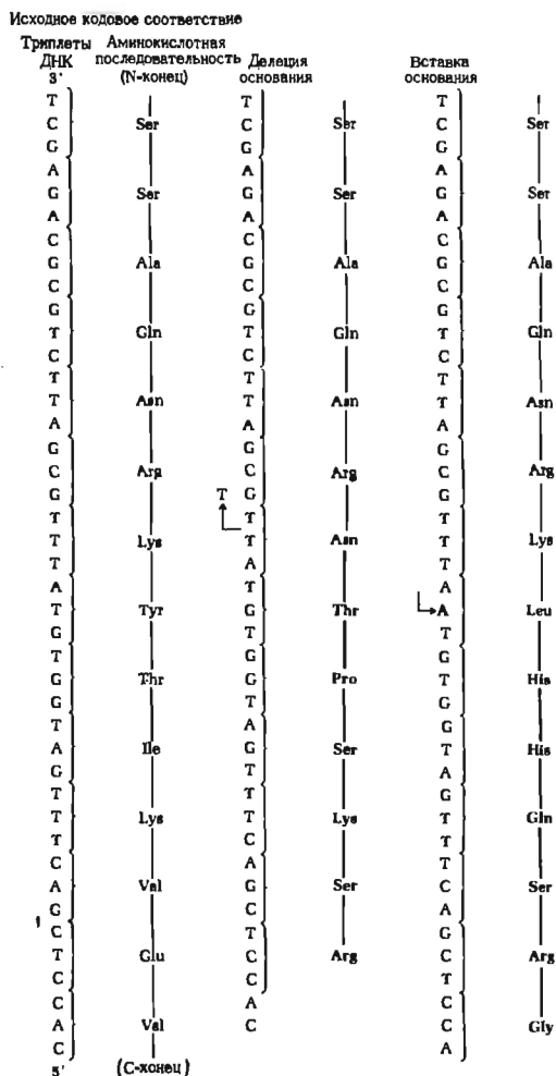
Рис. 30-8. Мутации со сдвигом рамки вызываются делецией или вставкой оснований (показаны красными стрелками). Начиная с кодона, в котором потеряно или приобретено основание, аминокислотная последовательность будет полностью искажена (изображена красным цветом). Большинство мутаций со сдвигом рамки летальны.
