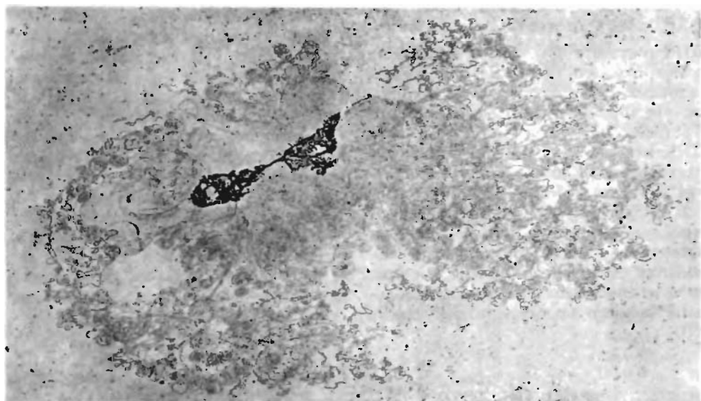
Рис. 27-19. Электронная микрофотография интактной сверхспиральной хромосомы, выделенной из одной клетки E. coli . Интактность хромосомы была установлена с помощью сильно увеличенной фотографии. Чуть влево от центра видны фрагменты клеточной мембраны.
