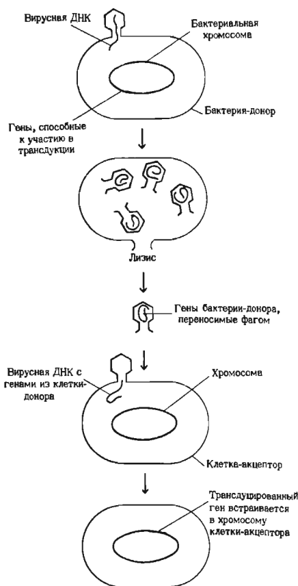
Рис. 30-12. Генетическая рекомбинация в ходе вирусной трансдукции бактериальных генов в реципиентную клетку.
