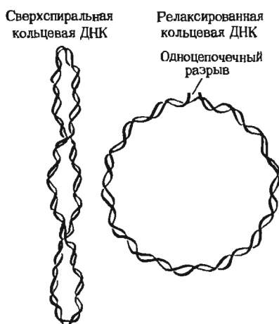
Рис. 27-18. Кольцевая сверхспиральная ДНК, закрученная в результате отрицательных поворотов, т.е. поворотов, противоположных по направлению к закручиванию самой двойной спирали. Разрыв одной из цепей такой ДНК снимает сверхспирализацию и приводит к переходу кольцевой ДНК в релаксированную форму.
