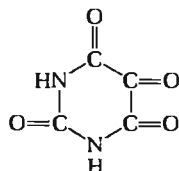
Рис. 25-18. Структура аллоксана — пиридинового производного, вызывающего экспериментальный диабет у животных путем разрушения островковых клеток.
