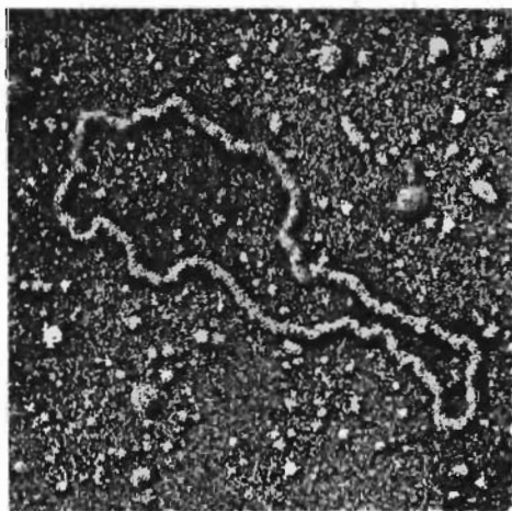
Рис. 27-20. Электронные микрофотографии плазмид, выделенных из двух видов бактерий. А. Плазмида pSC101 из E. coli , которая придает клеткам устойчивость к тетрациклину. Б. Плазмиды из Neisseria gonorrhoeae —бактерии, вызывающей гонорею. Большинство молекул находится в релаксированном состоянии. На примере скрученных сверхспиральных плазмид (одна из них в центре фотографии) видно, насколько эффективной может оказаться компактная упаковка кольцевой ДНК в результате отрицательных поворотов.
