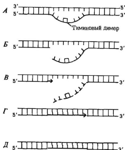
Рис. 30-2. А. Репарация тиминового димера. Б. Особая УФ-эндонуклеаза расщепляет дефектную цепь с 5'-стороны от димера. В. ДНК-полимераза I начинает «латать» цепь, а 5' → 3'-эндонуклеаза удаляет тиминовый димер и несколько прилежащих к нему нуклеотидов. Г. Новый участок ДНК построен. Д. Соединение нового участка с основной цепью под действием ДНК-лигазы.
