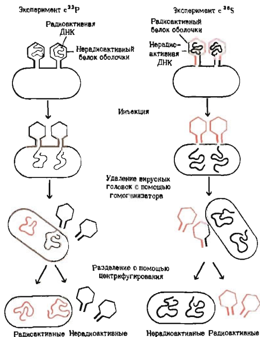
Рис. 27-7. Общая схема эксперимента Херши и Чейза. Эксперимент проводили на двух препаратах бактериофага, меченного радиоактивным изотопом. В одном из них с помощью изотопа ^{32}\text{P} были помечены фосфатные группы фажовой ДНК, а в другом изотоп ^{35}\text{S} был введен в серусодержащие аминокислоты белка оболочки фага. Каждый из меченных таким способом фагов по отдельности был добавлен к суспензии немеченых бактерий. Затем обе группы зараженных фагом бактериальных клеток встряхивали в смесителе. Оказалось, что клетки, зараженные ^{32}\text{P} -вирусными частицами, содержат в своем составе ^{32}\text{P} , т.е. в них попала меченая вирусная ДНК. Отделенные от клеток «тени» фага (пустые оболочки вируса) радиоактивности не содержали. В клетках, зараженных ^{35}\text{S} -вирусными частицами, радиоактивности не было, зато она была найдена в «тенях» фага после отделения их от клеток с помощью смесителя. Поскольку в обоих случаях было получено потомство вирусных частиц, данный эксперимент доказал, что генетическая информация, необходимая для репликации вируса, переносится вирусной ДНК, а не вирусным белком.
