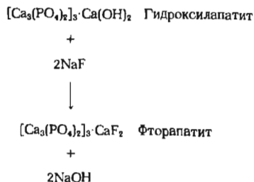
Рис. 26-28. Действие фторида натрия на гидроксилapatит.
