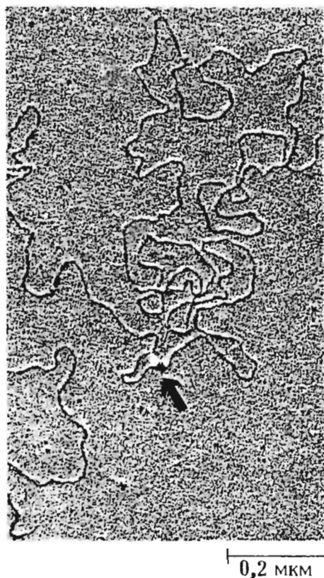
Рис. 29-26. Электронная микрофотография участка ДНК E. coli , на которой видна молекула lac -репрессора (указана стрелкой), присоединенная к lac -оператору.
