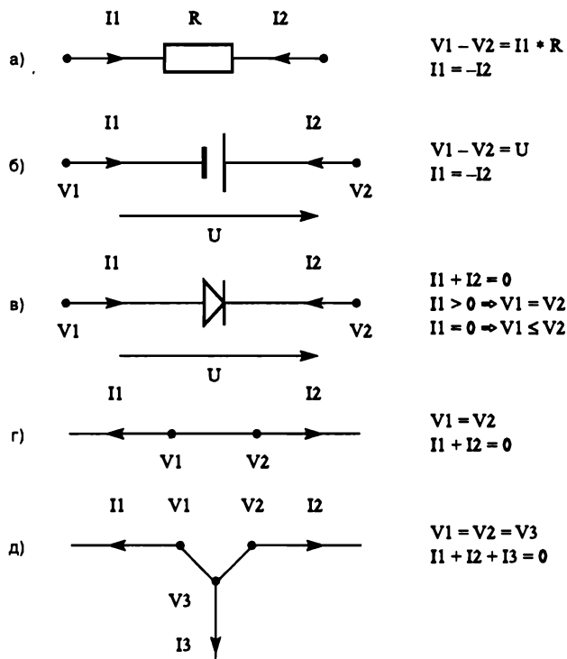
Рис. 14.3. Компоненты и соединения для электрических схем и соответствующие ограничения: а) резистор; б) источник питания; в) диод; г) соединение между двумя клеммами; д) соединение между тремя клеммами
