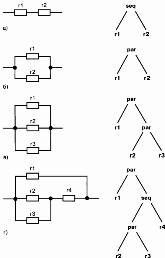
Рис. 2.6. Примеры простых электрических схем и их древовидных представлений: а) последовательное соединение резисторов r1 и r2; б) параллельное соединение двух резисторов; в) параллельное соединение трех резисторов; г) параллельное соединение резистора r1 и еще одной схемы
