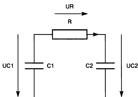
Рис. 20.7. Электрическая схема с двумя конденсаторами и резистором
