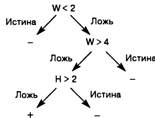
Рис. 18.3. Гипотеза 1, представленная в виде дерева решения. Внутренние узлы дерева обозначены атрибутами, листья — названиями классов, а ветви соответствуют значениям атрибутов. Например, самая левая ветвь соответствует W < 2 , а самый левый лист указывает, что соответствующий ему гриб является ядовитым (имеет класс “-”). Объект соответствует определенному листу, если он удовлетворяет всем условиям на пути от корня к данному листу
