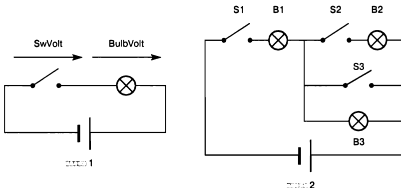
Рис. 20.2. Примеры простых схем, состоящих из выключателей, ламп и источников питания
