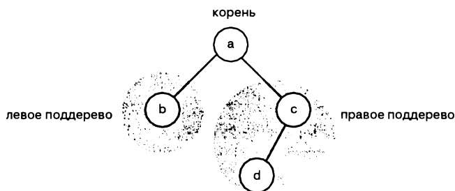
Рис. 9.2. Бинарное дерево
