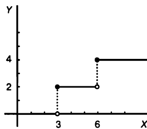
Рис. 5.1. Двухступенчатая функция
