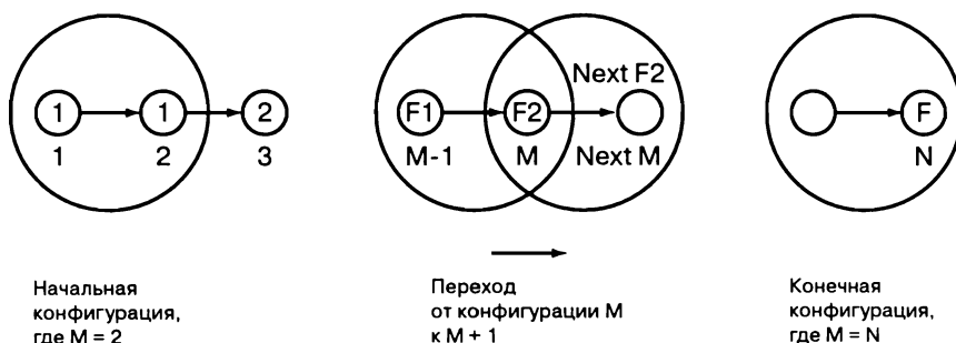
Рис. 8.4. Соотношения между числами ряда Фибоначчи; конфигурация, обозначенная большим кружком, определяется тремя компонентами: индексом M и двумя последовательными числами Фибоначчи, f(M-1) и f(M)
