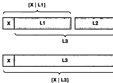
Рис. 3.2. Конкатенация списков
