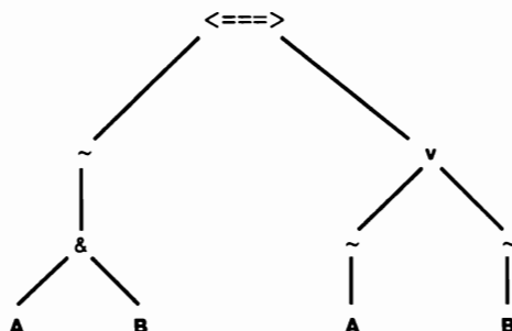
Рис. 3.8. Интерпретация терма \sim(A \& B) \<==> \sim A \vee \sim B
