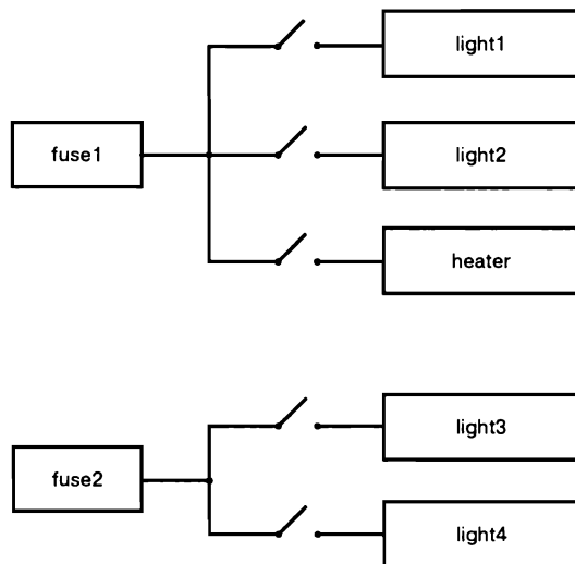
Рис. 16.1. Соединения между плавкими предохранителями и приборами в простой электрической сети
