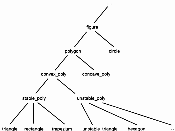
Рис. 18.6. Иерархия понятий
