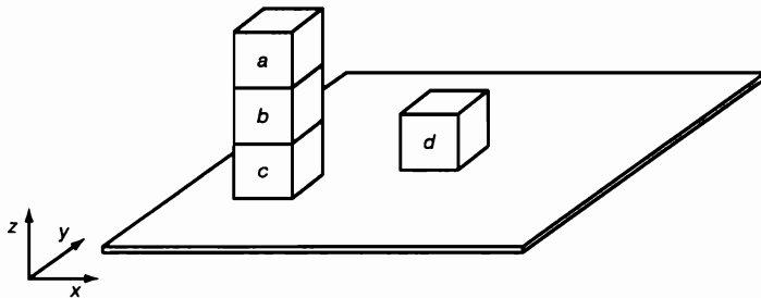
Рис. 23.1. Мир робота
