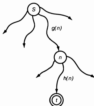
Рис. 12.1. Формирование эвристической оценки f(n) стоимости пути с наименьшей стоимостью от s до t через n : f(n) = g(n) + h(n)
