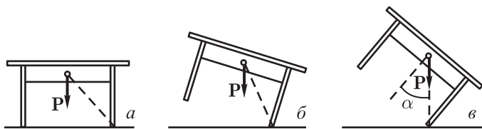
Рис. 134. При отклонении стола (б) от его положения равновесия (а) центр тяжести поднимается — равновесие устойчиво. В положении в) стол отклонен на предельный угол; при дальнейшем отклонении центр тяжести будет опускаться — равновесие неустойчиво
