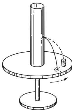
Рис. 392. При неподвижном столике струя воды из сосуда падает в стакан. При вращении столика струя воды падает сзади стакана
