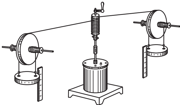
Рис. 365. Прибор Джоуля
