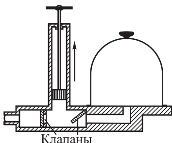
Рис. 280. Поршневой воздушный насос
