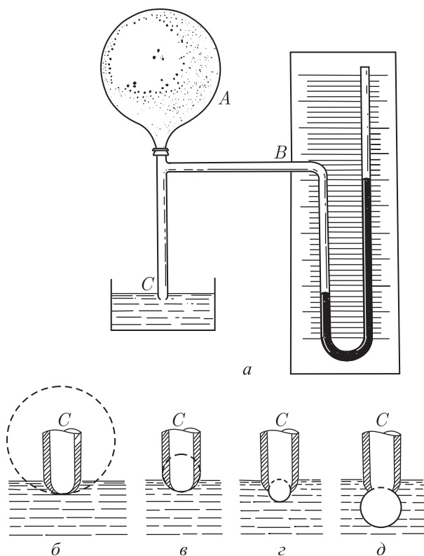
Рис. 419. a ) Прибор для выдувания пузырьков в жидкости. б)–г ) В начале выдувания пузырька радиус кривой поверхности жидкости постепенно уменьшается. д ) Под конец выдувания радиус поверхности снова увеличивается
