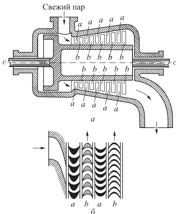
Рис. 515. а) Схема устройства паровой турбины. б) Расположение на валу cc турбины лопаток: a — направляющих, b — рабочих
