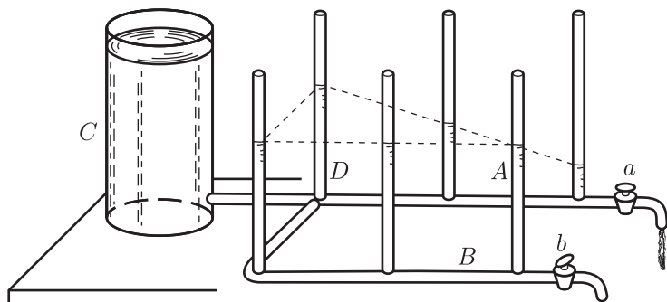
Рис. 310. Прибор для демонстрации падения давления в водопроводе
