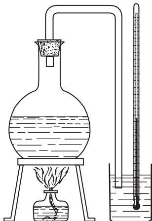
Рис. 488. Пока из кипятыльника идет воздух, термометр показывает почти одну и ту же температуру. Когда вместо воздуха пойдет пар и начнет конденсироваться в стаканчике столбик термометра быстро поднимется, показывая повышение температуры
