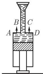
Рис. 253. При налипании воды в воронку цилиндр поднимается вверх
