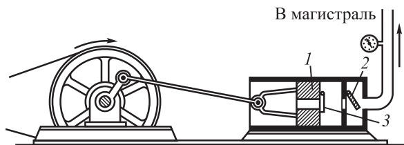
Рис. 302. Схема компрессора
