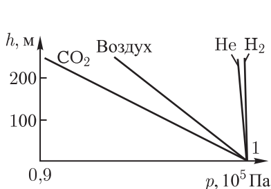
Рис. 297. Графики изменения давления p с высотой h для разных газов
