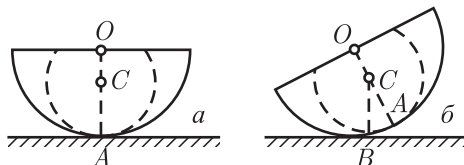
Рис. 133. Так как в положении а) центр тяжести расположен ниже, чем в положении б), то равновесие устойчиво
