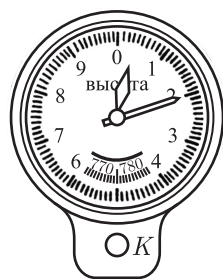
Рис. 295. Самолетный альтиметр. Длинная стрелка отсчитывает сотни метров, короткая — километры. Головка К позволяет подводить ноль циферблата под стрелку на поверхности Земли перед началом полета
