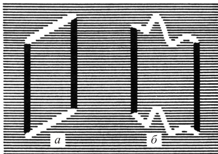
Рис. 7. Поступательное движение лунки
