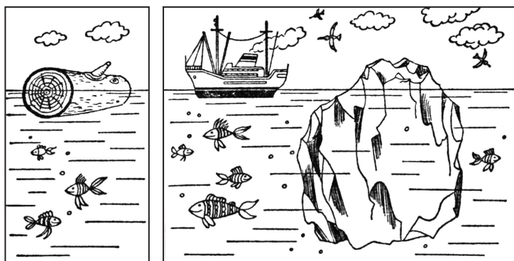
Рис. 265. Лыдина плавает, погрузившись в воду глубоко. Сосновое полено погружается при плавании только наполовину
