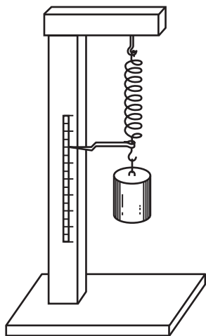
Рис. 58. Градуировка динамометра
