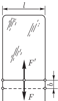
Рис. 405. Рамка, затянута мыльной пленкой
