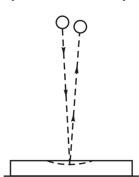
Рис. 168. Отразившись от стальной плиты, стальной шарик подскакивает снова почти на ту же высоту, с которой он был брошен
