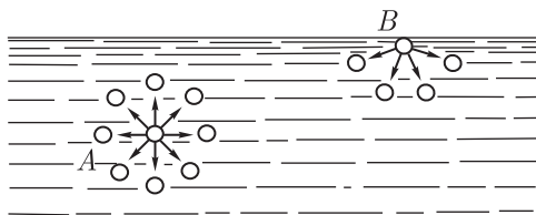
Рис. 398. Молекула A окружена со всех сторон другими молекулами и притягивается ими по всевозможным направлениям. Молекула B притягивается другими молекулами внутри жидкости
