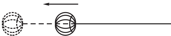
Рис. 167. Быстро летящий бумажный шарик растягивает резиновую нить
