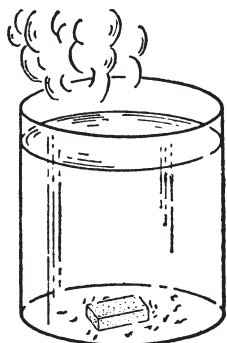
Рис. 457. Когда кипяток растворяет сахар, он сильно охлаждается
