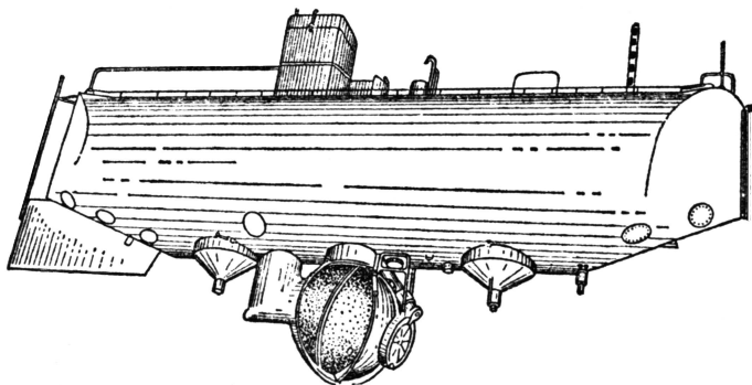
Рис. 254. Батискаф
