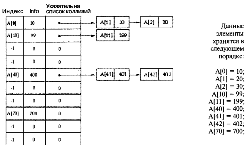
Рис. 4.2. Пример хэширования
