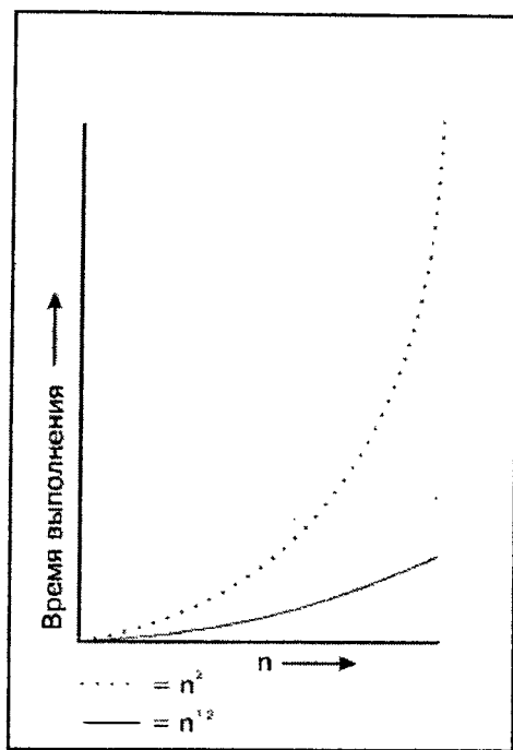
Рис. 1.3. Кривые n^2 и n^{1/2}
