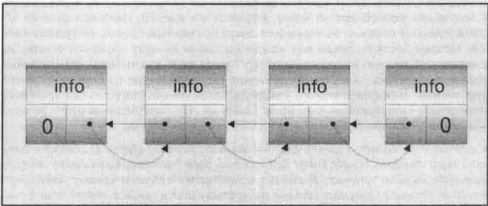
Рис. 2.1. Список с двойными связями
