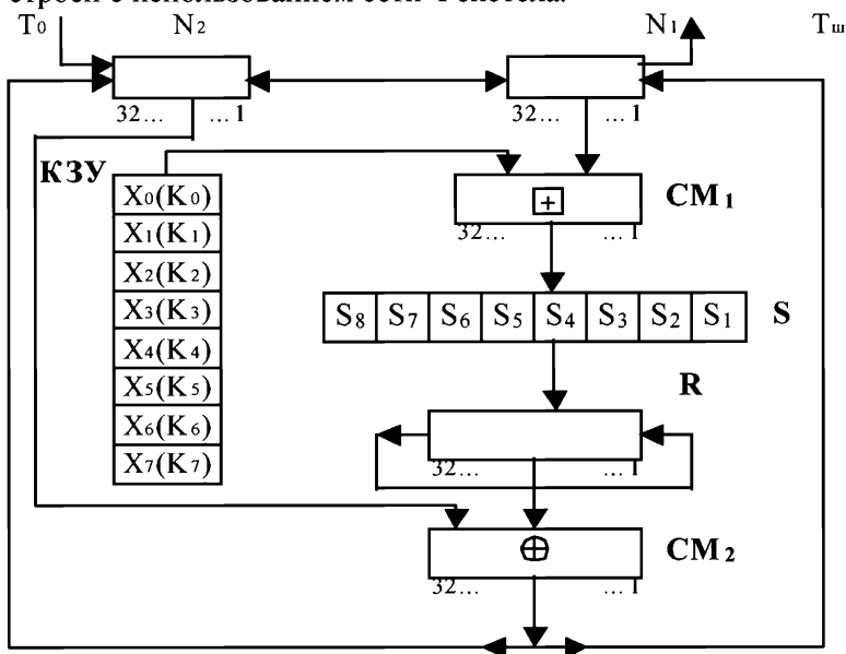
Рис 2.4. Алгоритм шифрования ГОСТ 28147-89.
