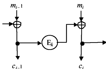
Рис. 2.7. Режим обратной связи по шифрованному тексту.
