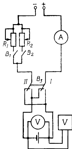
Рис. 37.3. Электрическая схема для заряда и разряда аккумулятора в широком диапазоне токовой нагрузки:
