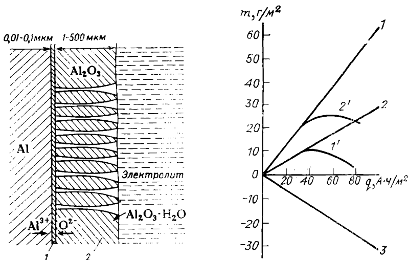
Рис. 13.1. Схема образования оксидной пленки на алюминии: 1 — плотная часть пленки; 2 — пористая часть пленки
