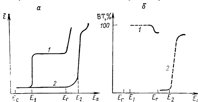
Рис. 11.1. Поляризационные кривые (а) и зависимость выхода по току (б) от потенциала: 1 — железо, никель в растворах \text{NaCl} ; 2 — железо, никель в растворах \text{NaNO}_3 ( \text{NaClO}_3 ); E_c — стационарный потенциал; E_1 — потенциал анодной активации в растворах \text{NaCl} ; E_2 — потенциал анодной активации в растворах \text{NaNO}_3 ( \text{NaClO}_3 ); E_f — потенциал начала газовой выделения.
