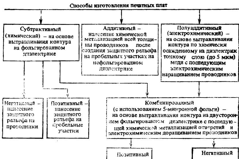
Рис. 16.1. Классификация способов изготовления печатных плат
