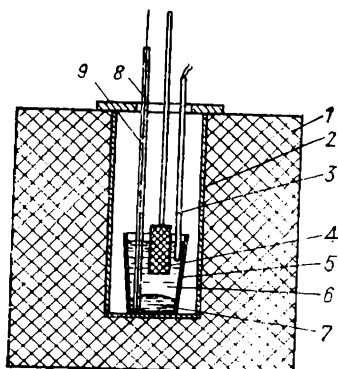
Рис. 22.1. Схема установки для получения тройного сплава:
