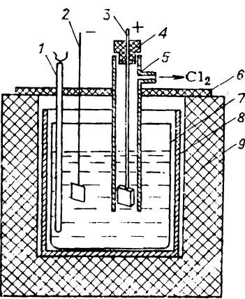
Рис. 23.1. Схема установки для получения магния:
