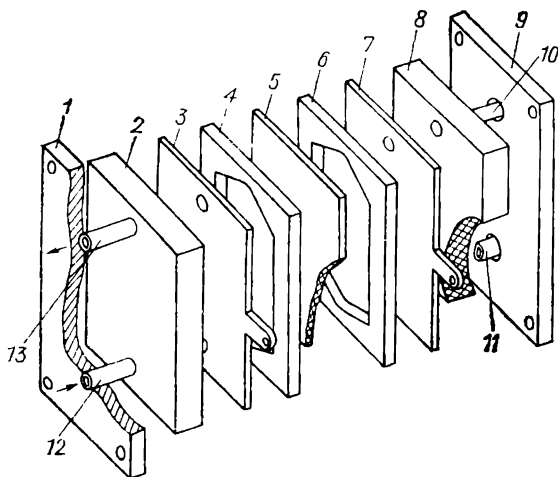
Рис. 27.5. Схема фильтр-прессного мембранного электролизера:
