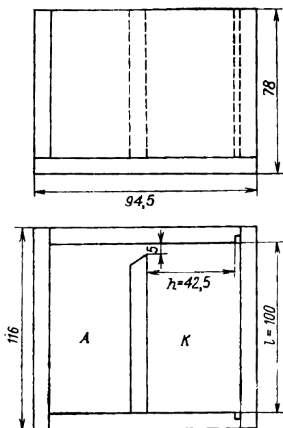
Рис. 1.1. Ячейка для измерения рассеивающей способности электролитов по ГОСТ 9.309—86:
