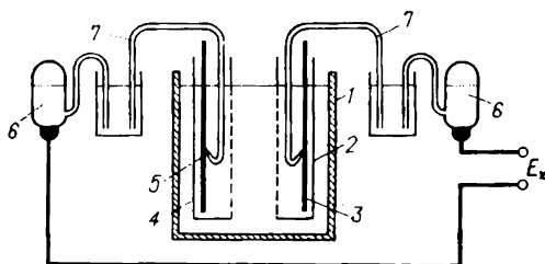
Рис. 25.1. Устройство ванны для электролиза воды с двумя электродными ячейками: 1—стеклянный корпус; 2—анодная ячейка; 3—катод; 4—катодная ячейка; 5—анод; 6—оксиднортутный электрод сравнения; 7—электролитический ключ с капилляром
