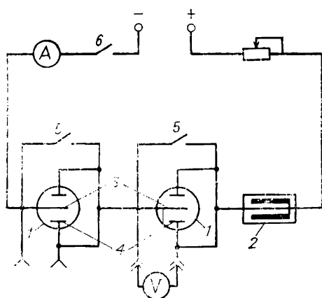
Рис. 1. Принципиальная схема установки для электролиза:
