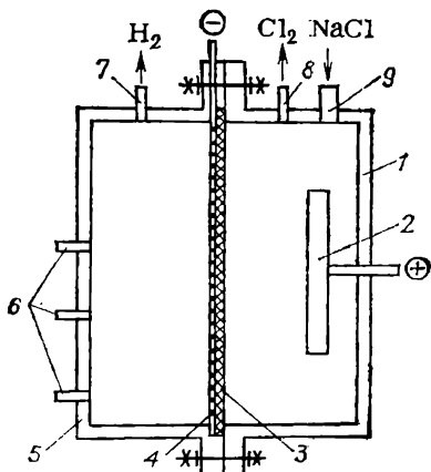
Рис. 27.3. Схема диафрагменного электролизера с плоскопараллельными вертикальными электродами:
