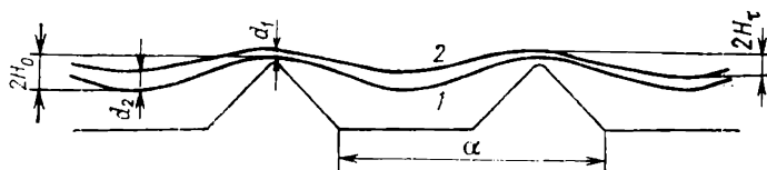
Рис. 2.2. Поперечный разрез двухслойного покрытия (слои 1 и 2), осажденного из выравнивающего электролита на поверхность с серией параллельных гребней треугольного поперечного сечения
