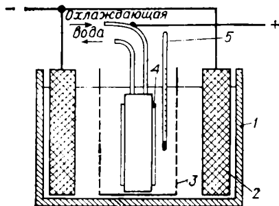
Рис. 29.1. Электролизер для получения персульфата аммония:
