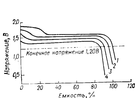
Рис. 37.1. Разрядные характеристики серебряно-цинкового аккумулятора в зависимости от тока нагрузки, кратного номинальной емкости C_{ном} :
