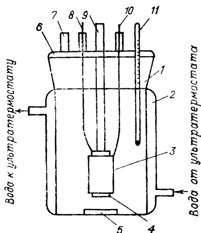
Рис. 33.1. Электролизер для электроокисления спиртов:
