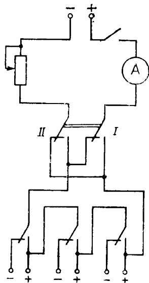
Рис. 34.2. Электрическая схема зарядно-разрядного стенда для группового циклирования аккумуляторов
