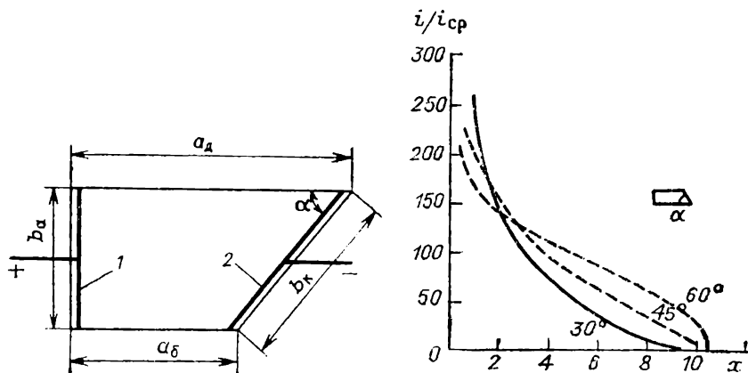
Рис. VII. Схема ячейки Хуллы:
