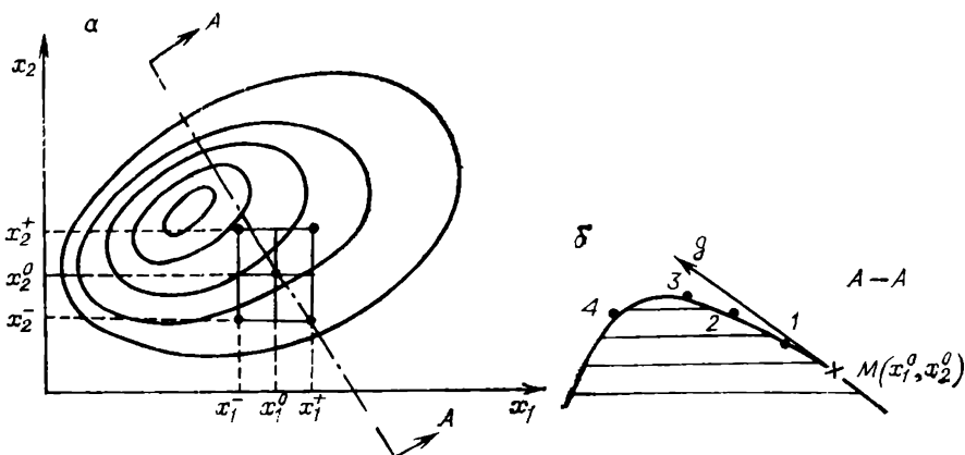
Рис. 18.1. Поиск экстремума методом крутого восхождения:
