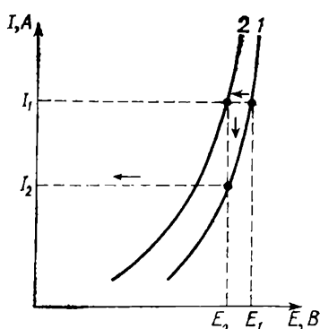
Рис. 26.3. Поляризационные кривые биполярного электрода, позволяющие рассчитать утечку тока:
