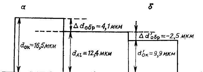
Рис. 13.3. Рассчитанные для q = 100 \text{ А} \cdot \text{ч}/\text{м}^2 объемные изменения при анодировании: а — d_{\text{ок}} и d_{\text{ок}\delta\text{р}} , если пленка не растворяется; б — d_{\text{ок}} и d_{\text{ок}\delta\text{р}} , если растворится 4% пленки
