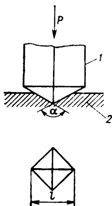
Рис. V. Схема измерения микротвердости
