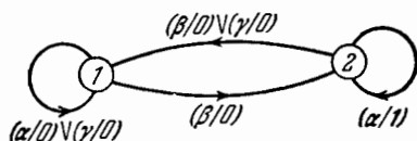
Рис. 7.5. Автомат АЗЗ.
