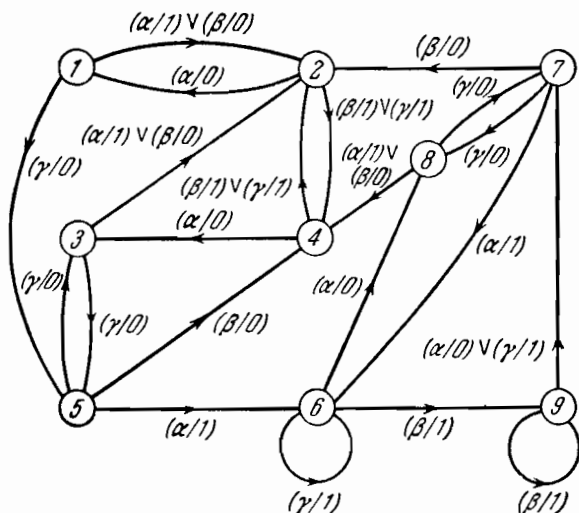
Рис. 3.3. Автомат A_7 .
