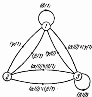
Рис. 7.2. Автомат A\check{3}2_1 .
