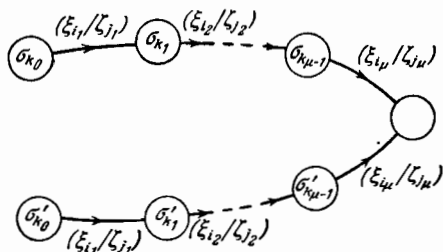
Рис. 6.3. (\xi_{i_1}|\zeta_{j_1})(\xi_{i_2}|\zeta_{j_2}|\zeta_{j_\mu}) -совпадающие пути.
