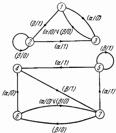
Рис. 2.8. Автомат Δ (A4, A5).
