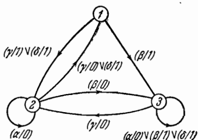
Рис. 7.3. Автомат A\check{3}2_2 .
