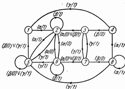
Рис. 3.1. Автомат А6.
