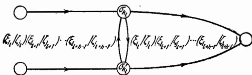
Рис. 6.5. Иллюстрация доказательства теоремы 6.1.
