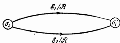
Рис. 5.4. Состояние с потерей информации.
