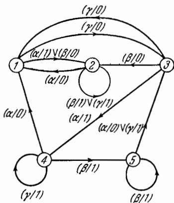
Рис. 3.9. Автомат \check{A}7 .
