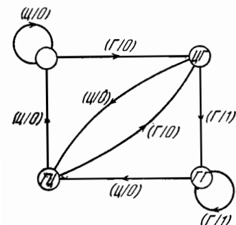
Рис. 3.10. Автомат A15.
