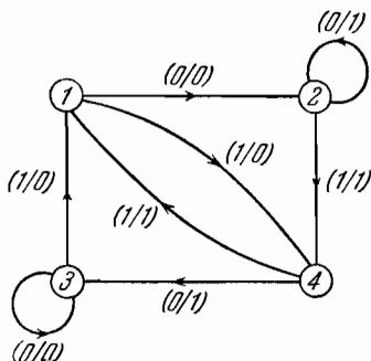
Рис. 6.2. Автомат A27.
