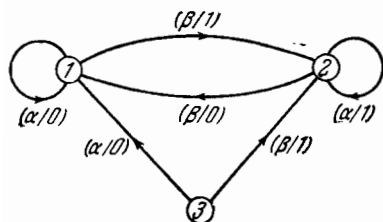
Рис. 3.7. Автомат A_{10} .
