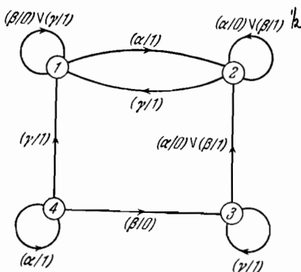
Рис. 3.12. Автомат A6 .
