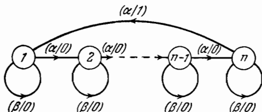
Рис. 4.4. Автомат A18.
