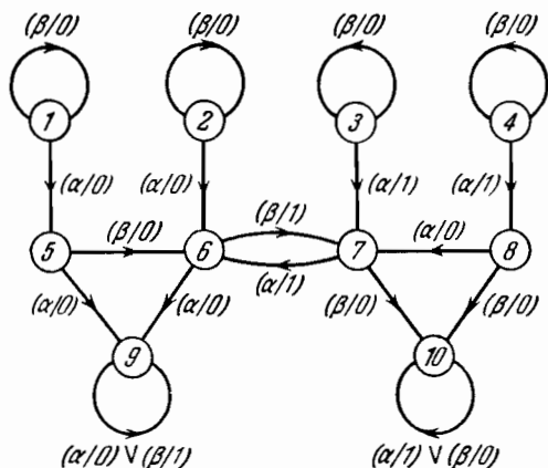
Рис. 4.10. Автомат \dot{A}21 .
