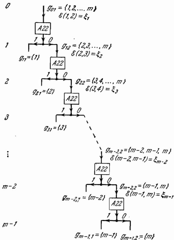
Рис. 4.14. Дерево кратного эксперимента для A22 и множества допустимых начальных состояний \{1, 2, \dots, m\} .
