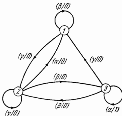
Рис. 7.4. Автомат А33.
