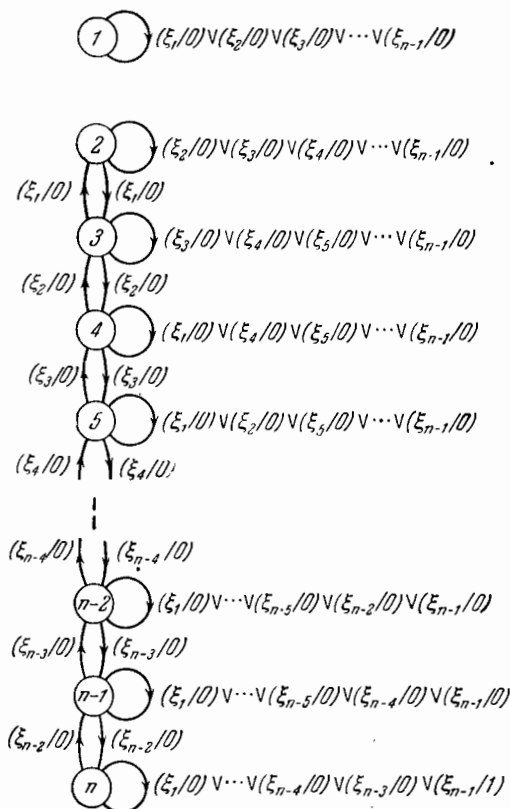
Рис. 4.17. Автомат M^* .
