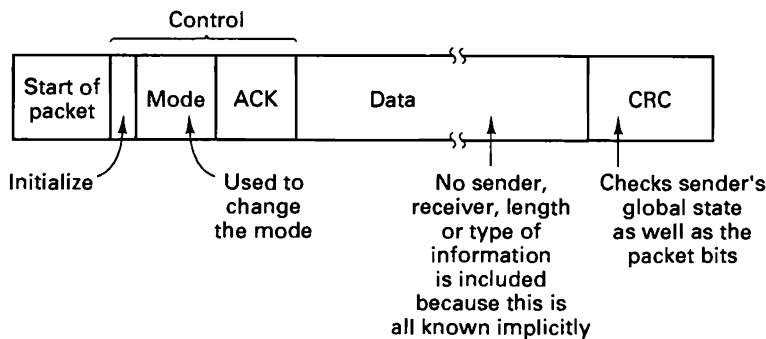
Fig. 4-29. A typical TTP packet.
