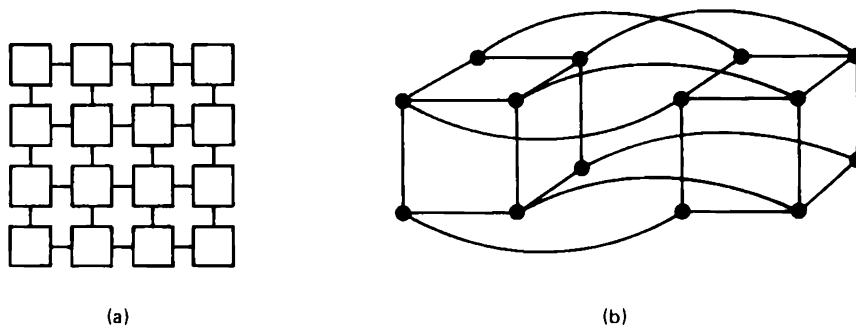
Fig. 1-8. (a) Grid. (b) Hypercube.
