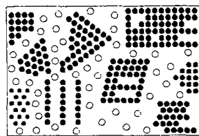
Рис. 5.5. Схематическое изображение строения нанокристаллического материала; ● — атомы нанокристалла, ○ — атомы, находящиеся на границах между нанокристаллами.
