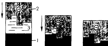
Рис. 38.4. Электрохимическое объемное копирование: 1 — анод; 2 — катод; 3 — электролит.
