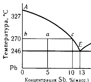
Рис. 12.8. Часть диаграммы состояния системы Pb—Sb.
