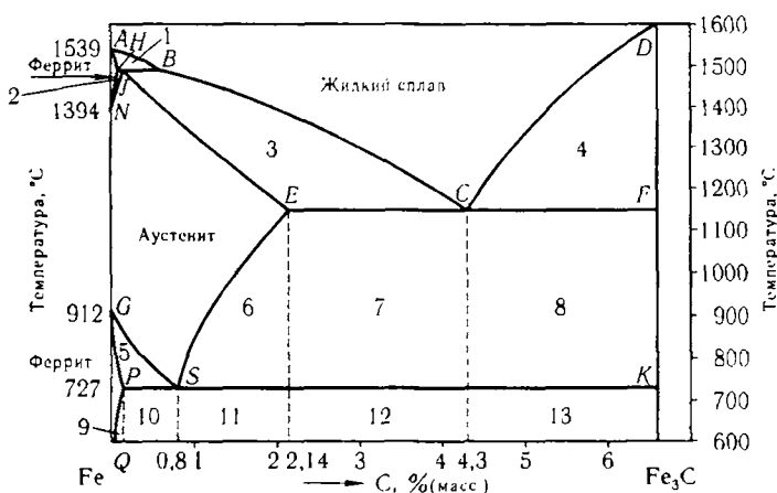
Рис. 32.2. Диаграмма состояния системы железо—углерод
