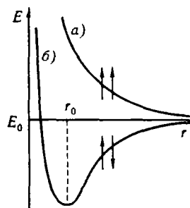
Рис. 4.1. Зависимость энергии системы, состоящей из двух атомов водорода от межатомного расстояния: a — при одинаково направленных спинах электронов; b — при противоположно направленных спинах; E_0 — энергия системы из двух невзаимодействующих атомов водорода; r_0 — равновесное межъядерное расстояние в молекуле водорода.
