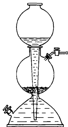
Рис. 19.1. Аппарат Киппа.
