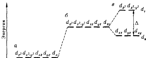
Рис. 13.2. Схема энергетических уровней d -орбиталей центрального иона: а — свободный ион; б — ион в гипотетическом сферическом поле; в — ион в октаэдрическом поле лигандов.
