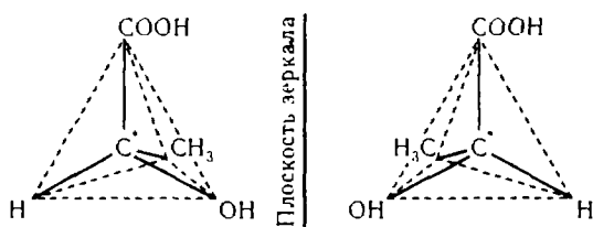
Рис. 29.11. Тетраэдрические модели молекул зеркальных изомеров молочной кислоты.
