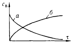
Рис. 6.6. Изменение концентрации исходного вещества (а) и продукта реакции (б) со временем.
