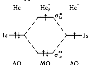
Рис. 4.9. Схема МО молекулярного иона гелия.
