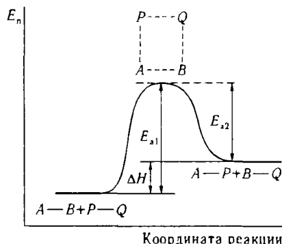
Рис. 6.8. Изменение потенциальной энергии между реакционными центрами в бимолекулярной реакции: AB и PQ — исходные вещества; AP и BQ — продукты реакции; APQV — переходное состояние; E_{a1} — энергия активации прямой реакции; E_{a2} — энергия активации обратной реакции; \Delta H — тепловой эффект реакции.
