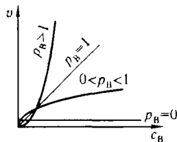
Рис. 6.13. Влияние порядка реакции на изменение скорости реакции v = kc_A^{p_A} c_B^{p_B} .
