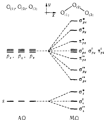
Рис. 18.3. Приближенная схема МО озона.
