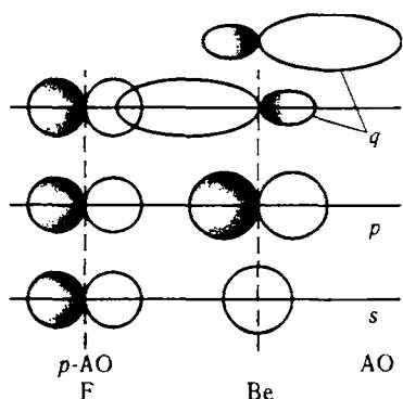
Рис. 4.27. Схема перекрывания p -АО фтора и s -, p - и гибридной q(sp) -АО бериллия. Одна гибридная орбиталь бериллия для наглядности показана смещенной вверх от общей оси.
