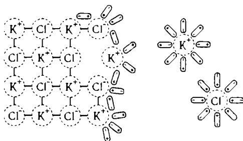
Рис. 8.1. Схема растворения соли.
