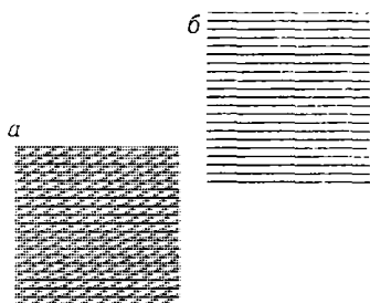
Рис. 4.45. Схема заполнения электронами энергетических уровней в кристалле элемента главной подгруппы второй группы: а — валентная зона, образованная из исходных внешних s -орбиталей; б — зона проводимости, образованная из исходных внешних p -орбиталей.
