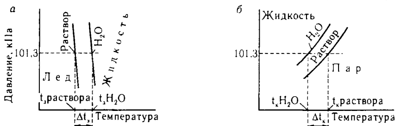
Рис. 7.8. Часть диаграммы состояния воды и раствора в области давлений, близких к 101,3 кПа: а — кривые плавления; б — кривые кипения.
