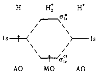
Рис. 4.8. Схема МО молекулярного иона водорода.
