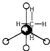
Рис. 29.3. Шариковая модель молекулы метана.
