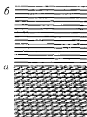
Рис. 4.44. Схема заполнения электронами энергетических уровней в кристалле щелочного элемента: а — занятые уровни (валентная зона), б — незанятые уровни (зона проводимости).
