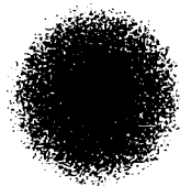
Рис. 2.5. Электронное облако атома водорода.
