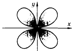
Рис. 2.18. Схематическое изображение типичного электронного облака 3d -электрона.
