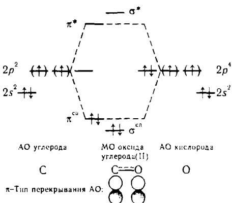
Рис. 4.16. Образование \pi -МО из АО неспаренных электронов.
