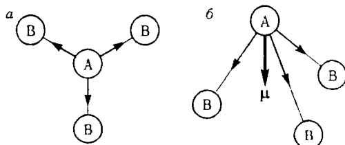
Рис. 4.33. Дипольные моменты отдельных связей и молекул AB_3 : а — плоский треугольник; б — пирамида; \mu — вектор суммарного дипольного момента молекулы.
