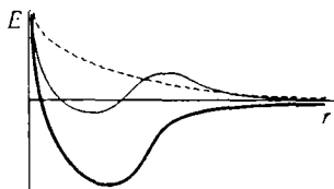
Рис. 4.46. Характер изменения энергии взаимодействия двух молекул от расстояния между ними: жирная кривая показывает притяжение молекул в начале сближения, а затем их отталкивание; обычная кривая — сначала отталкивание молекул, а затем притяжение и потом вновь отталкивание; штриховая кривая отвечает постоянному отталкиванию.
