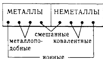
Рис. 12.1. Положение элемента среди металлов и неметаллов и вид химической связи в бинарном соединении.
