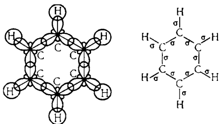
Рис. 29.12. Схема образования \sigma -связей в молекуле бензола.
