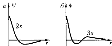
Рис. 2.12. Волновые функции для 2s - (а) и 3s -электронов (б).
