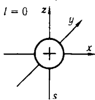
Рис. 2.20. Ориентация и форма s-АО: s-АО симметрична по отношению к основным операциям точечной группы симметрии: вращению, отражению и инверсии.
