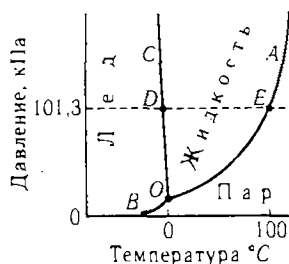
Рис. 7.2. Диаграмма состояния воды в области невысоких давлений.
