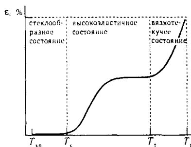
Рис. 31.2. Изменение относительных размеров образца полимера ( \epsilon ) при действии постоянной нагрузки в зависимости от температуры: T_{хр} — температура хрупкости, T_c — температура стеклования (размягчения), температура текучести, T_p — температура разложения.
