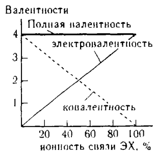
Рис. 9.1. Изменение ковалентности и электровалентности центрального атома идеализированной молекулы состава ЭХ 4 в зависимости от ионности химической связи; атом Х одновалентный атом, типа Н, F и т. п.
