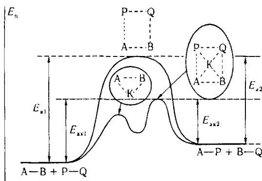
Рис. 6.16. Энергетическая схема реакции, протекающей с участием катализатора: АВ и PQ — исходные вещества; AP и BQ — продукты реакции; APQB — переходное состояние без катализатора; ABK — первое переходное состояние в присутствии катализатора; ABPQK — второе переходное состояние в присутствии катализатора; E_{a1} — энергия активации прямой реакции без катализатора; E_{a2} — энергия активации обратной реакции без катализатора; E_{ак1} — энергия активации прямой реакции в присутствии катализатора; E_{ак2} — энергия активации обратной реакции в присутствии катализатора.
