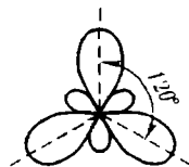
Рис. 4.28. Взаимное расположение гибридных sp^2 -орбиталей.
