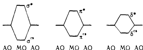
Рис. 4.13. Расщепление энергий МО различной симметрии.
