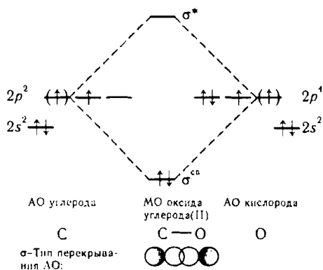
Рис. 4.15. Образование \sigma -МО из АО неспаренных электронов.
