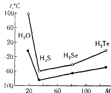
Рис. 4.48. Зависимость температуры плавления (●) и кипения (○) водородных соединений элементов главной подгруппы VI группы от молекулярной массы.
