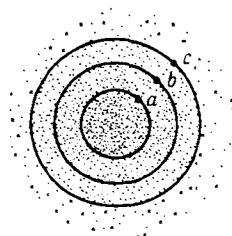
Рис. 2.8. К понятию о размерах и форме электронного облака.
