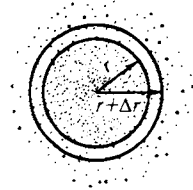
Рис. 2.10. Электронное облако 1s -электрона.
