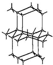
Рис. 7.1. Структура льда.
