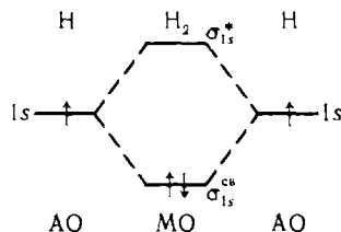
Рис. 4.7. Схема МО молекулы водорода.
