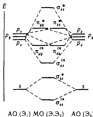
Рис. 4.22. Схема образования МО из АО в двухатомных молекулах \mathcal{E}_1\mathcal{E}_2 .
