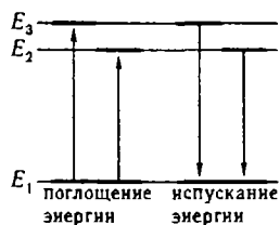
Рис. 2.4. К происхождению линейчатых спектров поглощения и испускания.
