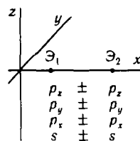
Рис. 4.21. Расположение атомов молекулы \text{Э}_1\text{Э}_2 в декартовой системе координат и типы попарно наиболее эффективно взаимодействующих АО.
