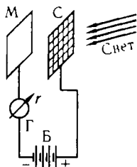
Рис. 2.3. Схема установки для наблюдения фотоэлектрического эффекта:
