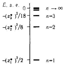
Рис. 2.6. Энергии электронных оболочек атома.
