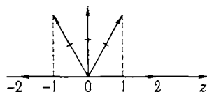
Рис. 2.19. К возможному набору значений магнитного квантового числа. Стрелками показаны допустимые направления орбитального момента количества движения.
