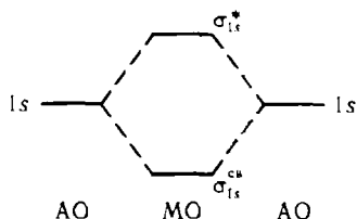
Рис. 4.6. Схема МО при взаимодействии идентичных 1s -АО.
