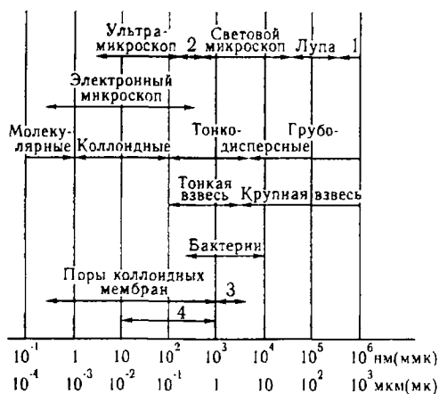
Рис. 10.7. Границы размеров частиц дисперсных систем и применения оптических методов определения дисперсности: 1 — глаз; 2 — ультрафиолетовый микроскоп. Для сравнения показан размер пор бумажных фильтров (3) и пор ультрафильтров (4).
