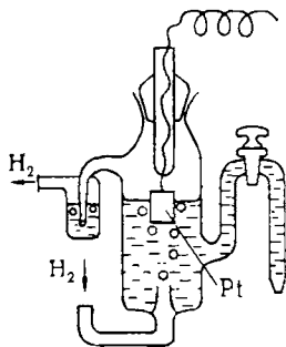
Рис. 9.5. Водородный электрод.
