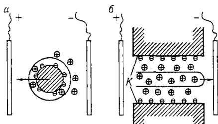
Рис. 10.15. Схема передвижения коллоидной частицы при электрофорезе (а) и электроосмотического переноса жидкости через капилляр (б) ( K — внутренняя поверхность капилляра). Поверхности коллоидной частицы и капилляра заряжены отрицательно.
