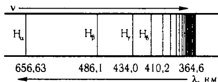
Рис. 2.2. Линейчатый спектр атома водорода в видимой и близкой ультрафиолетовой области (серия Бальмера); \lambda — длина волны, \nu — частота.
