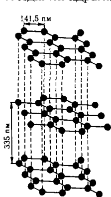
Рис. 16.2. Структура графита.
