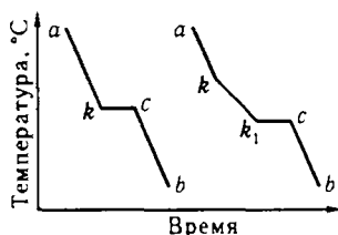
Рис. 12.4. Кривые охлаждения.
