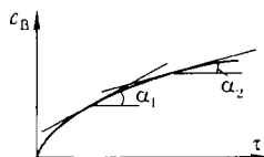
Рис. 6.7. Графическое определение скорости реакции: \operatorname{tg} \alpha_1 > \operatorname{tg} \alpha_2 , v_1 > v_2 .
