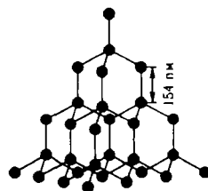
Рис. 16.1. Структура алмаза.
