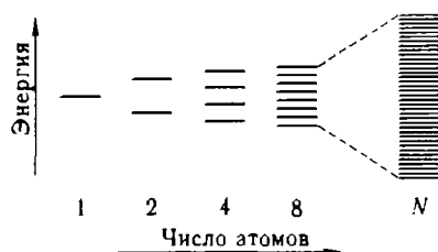
Рис. 4.43. Схема образования энергетических уровней МО при увеличении числа взаимодействующих атомов.
