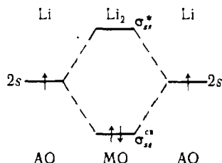
Рис. 4.20. Схема МО молекулы лития \text{Li}_2 .
