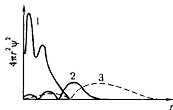
Рис. 2.23. Радиальное распределения вероятности нахождения электронов в атоме натрия. 1 — для десяти электронов K - и L -слоев; 2 — для 3s -электронов; 3 — для 3p -электронов.
