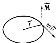
Рис. 2.7. К понятию об орбитальном моменте количества движения.
