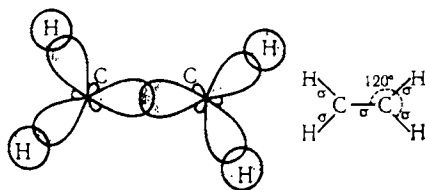
Рис. 29.6. Схема образования \sigma -связей в молекуле этилена.
