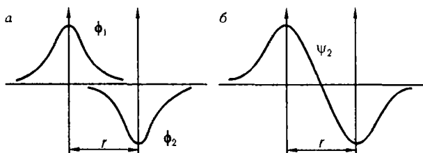
Рис. 4.5. Схема образования разрыхляющей МО из атомных 1s -орбиталей.
