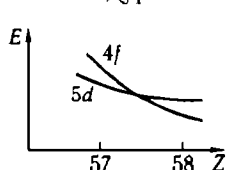
Рис. 2.24. Зависимость энергии 4f - и 5d -электронов от заряда ядра Z .
