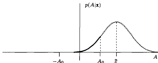
(b) \bar{x} > A_0
