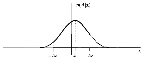
(a) -A_0 \leq \bar{x} \leq A_0
