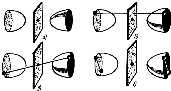
Рис. 59. а) тождественное преобразование; б) отражение в плоскости yz ; в) отражение в точке O ; г) отражение в плоскости ux
