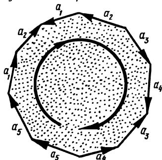
Рис. 105. W = a_1 a_2 a_1^{-1} a_2^{-1} a_3 a_4 a_3^{-1} a_4^{-1} a_5 a_5
