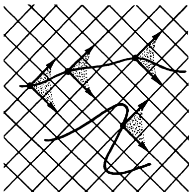
Рис. 17. Мировой линии, изображенной в нижней части рисунка быть не может
