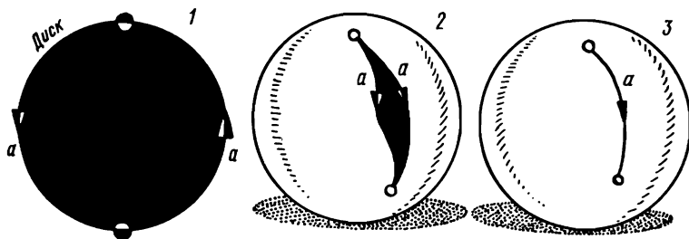
Рис. 112. W = aa^{-1} — не триангуляция
