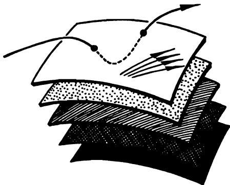
Рис. 64. Такой интегральной траектории быть не может
