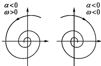
Рис. 123. Устойчивые фокусы
