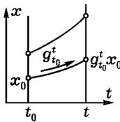
Рис. 70. Преобразование за время от t_0 до t
