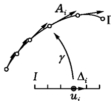
Рис. 8. Определение интеграла 1-формы
