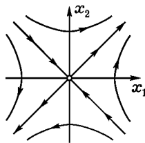
Рис. 33. Фазовые кривые перевернутого маятника
