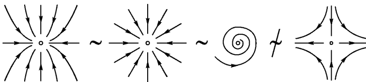
Рис. 151. Топологически эквивалентные и неэквивалентные системы
