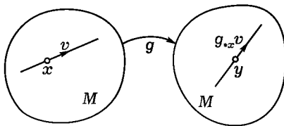
Рис. 57. Действие диффеоморфизма на поле направлений
