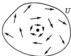
Рис. 164. Останутся ли вблизи положения равновесия фазовые кривые, начинающиеся в его достаточно малой окрестности?
