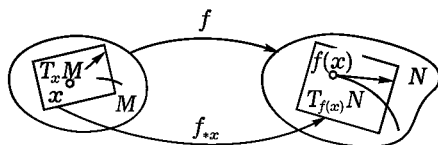
Рис. 255. Производная отображения f в точке x
