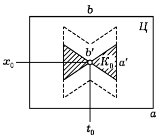
Рис. 221. Цилиндр \Pi и конус K_0
