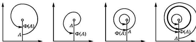
Рис. 17. Функция последования
