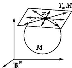
Рис. 249. Касательное пространство
