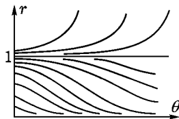
Рис. 55. Интегральные кривые на плоскости (r, \theta)
