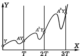
Рис. 41. Оператор монодромии
