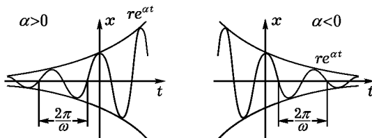
Рис. 126. Вещественная часть e^{\lambda t} как функция времени
