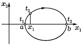
Рис. 103. Половину фазовой кривой (от a до b ) фазовая точка проходит за конечное время T/2 = t_2 - t_1
