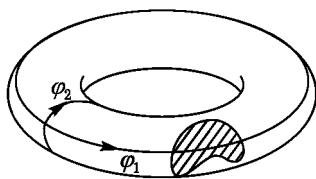
Рис. 172. Тор
