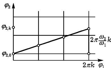
Рис. 178. Редукция теоремы к лемме
