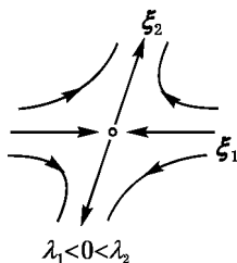
Рис. 134. Седло
