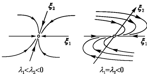
Рис. 133. Устойчивые узлы
