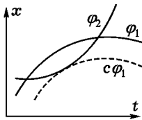
Рис. 77. Невозможное расположение графиков
