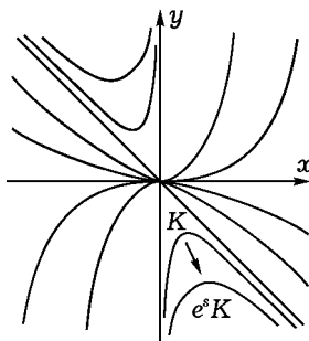
Рис. 65. Интегральные кривые однородного уравнения
