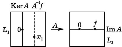
Рис. 183. Ядро и образ оператора A
