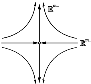
Рис. 162. Стандартное седло
