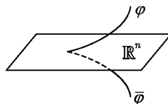
Рис. 128. Решение с вещественным начальным условием не может принимать комплексных значений
