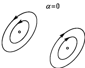
Рис. 137. Центры
