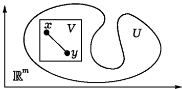
Рис. 220. Из непрерывной дифференцируемости вытекает выполнение условия Липшица
