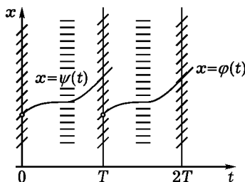
Рис. 204. Расширенное фазовое пространство уравнения с периодическими коэффициентами
