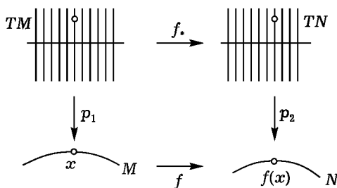
Рис. 256. Касательное отображение
