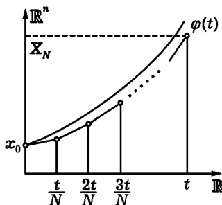
Рис. 111. Ломаная Эйлера
