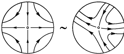
Рис. 152. Топологическая эквивалентность системы и ее линеаризации
