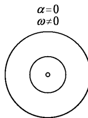
Рис. 125. Центр
