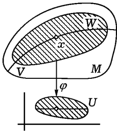
Рис. 246. Подмногообразие
