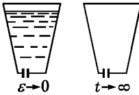
Рис. 71. Асимптотическое поведение решений возмущенного уравнения
