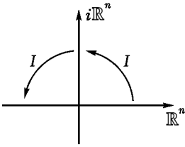
Рис. 117. Оператор умножения на i
