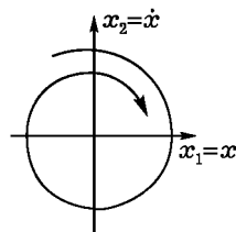
Рис. 139. Фазовая плоскость маятника с малым трением
