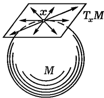
Рис. 49. Касательное пространство
