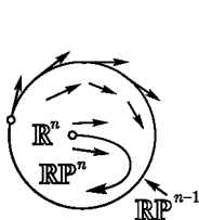
Рис. 260. Продолжение линейного векторного поля на проективное пространство
