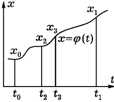
Рис. 28. Доказательство единственности
