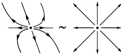
Рис. 154. Все неустойчивые узлы топологически эквивалентны
