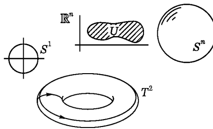
Рис. 231. Примеры многообразий
