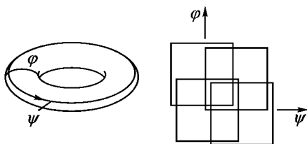
Рис. 236. Атлас тора
