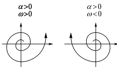
Рис. 124. Неустойчивые фокусы
