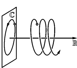
Рис. 121. Фазовая и интегральная кривые уравнения \dot{z} = \lambda z при чисто мнимом \lambda
