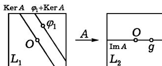
Рис. 43. Пространство решений линейного неоднородного уравнения
