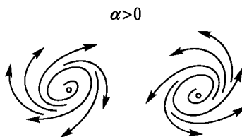
Рис. 138. Неустойчивые фокусы
