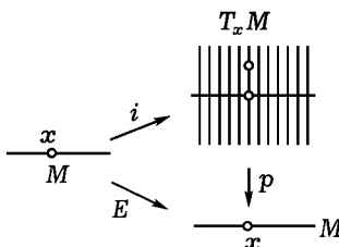
Рис. 251. Касательное расслоение
