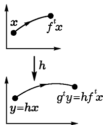
Рис. 149. Эквивалентные потоки
