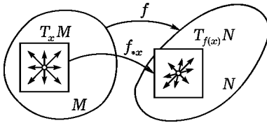
Рис. 52. Производная отображения в точке
