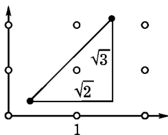
Рис. 179. Фазовая кривая системы \dot{\varphi}_1 = 1, \dot{\varphi}_2 = \sqrt{2}, \dot{\varphi}_3 = \sqrt{3} всюду плотна на трехмерном торе
