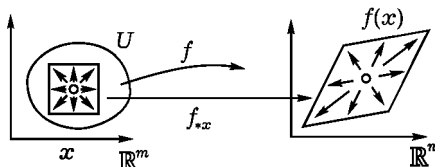
Рис. 219. Производная отображения f
