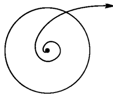
Рис. 157. Положительная определенность формы (4) в случае n = 1
