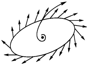
Рис. 155. Поверхность уровня функции Ляпунова
