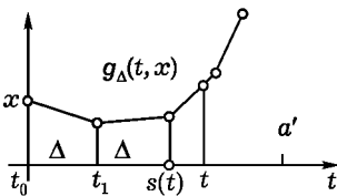
Рис. 224. Ломаная Эйлера
