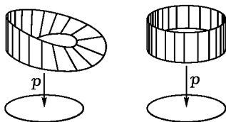
Рис. 253. Расслоение, не являющееся прямым произведением
