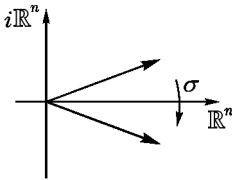
Рис. 118. Комплексное сопряжение
