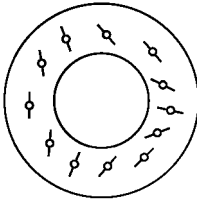
Рис. 58. Поле направлений, не достраиваемое до векторного поля
