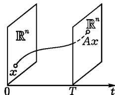
Рис. 205. Отображение монодромии
