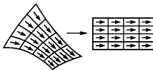
Рис. 74. Выпрямление векторного поля
