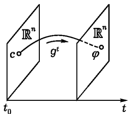
Рис. 210. Координаты точки c являются первыми интегралами однородного уравнения
