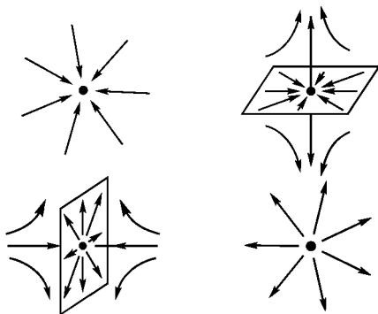
Рис. 163. Усы трехмерных седел
