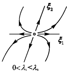
Рис. 135. Неустойчивый узел
