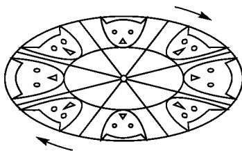
Рис. 132. Эллиптический поворот
