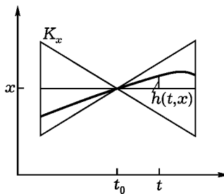
Рис. 222. Определение h(t, x)
