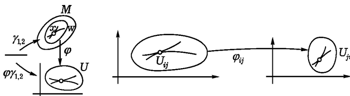
Рис. 248. Касательный вектор
