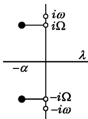
Рис. 187. Собственные числа уравнения маятника с трением
