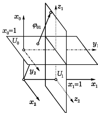
Рис. 237. Аффинные карты проективной плоскости
