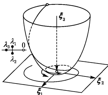
Рис. 147. Случай \lambda_3 < \operatorname{Re} \lambda_{1,2} < 0 . Сжатие по направлению \xi_3 , вращение с более медленным сжатием в плоскости (\xi_1, \xi_2)
