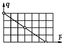
Рис. 68. Диаграмма Ньютона квазиоднородной функции
