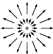
Рис. 61. Эйлерово поле
