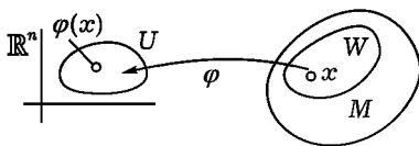
Рис. 232. Карта
