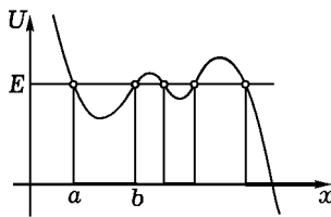
Рис. 100. Множество точек x , где U(x) < E
