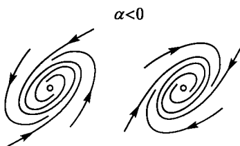
Рис. 136. Устойчивые фокусы
