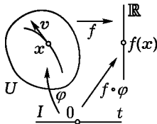
Рис. 84. Производная функции f по направлению вектора \mathbf{v}
