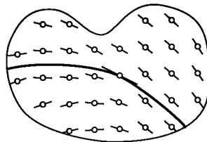
Рис. 3. Поле направлений и его интегральная кривая
