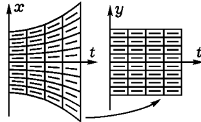
Рис. 69. Выпрямление поля направлений
