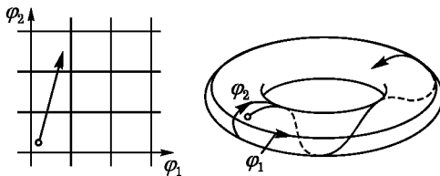
Рис. 174. Обмотка тора
