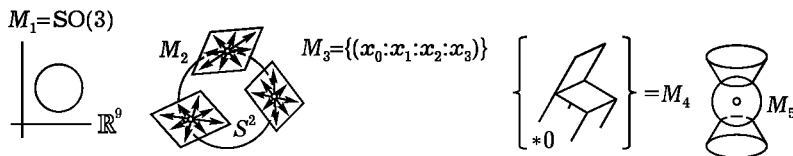
Рис. 247. Примеры трехмерных многообразий
