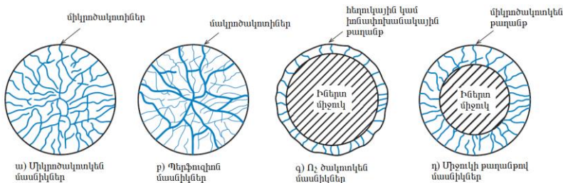
Նկար 11. Բարձրադրույունավետ հեղուկային քրոմատոգրաֆիայում կիրառվող մասնիկների կառուցվածքների տեսակները
