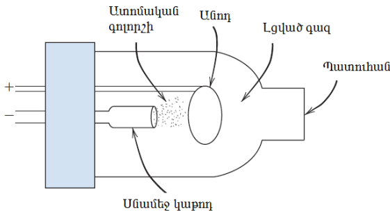
Նկար 20. Սնամեջ կաթոդային լամպի կառուցվածքը
