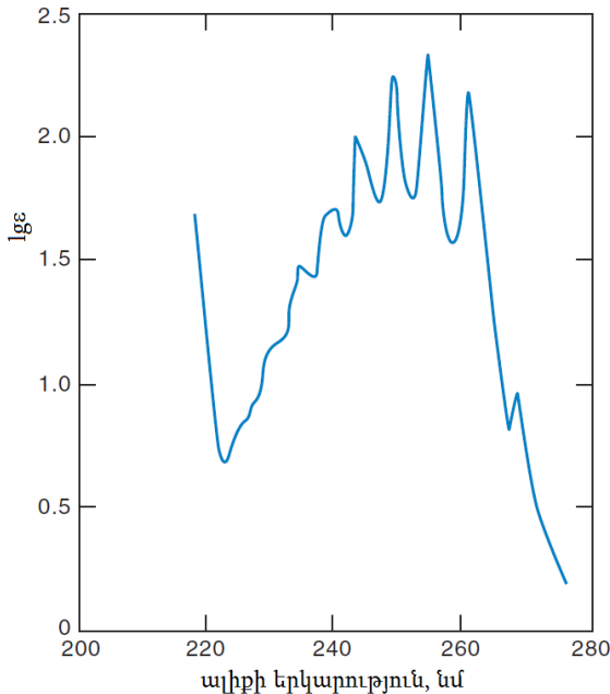
Նկար 3. Քենզոլի էլեկտրոնային կլանման սպեկտրը
