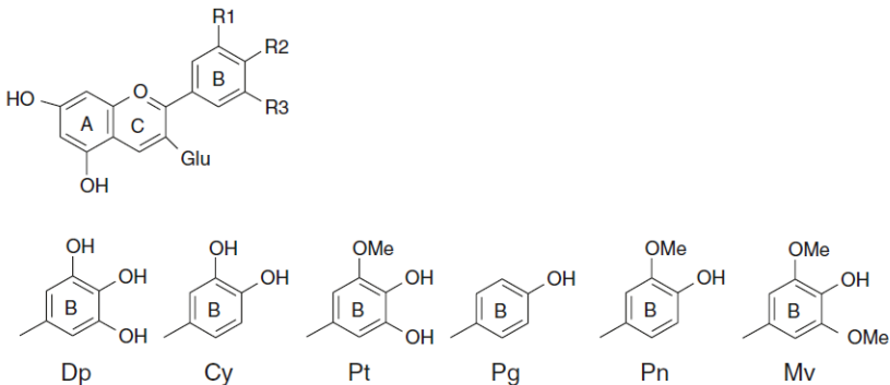
Նկար 17. Անտոցիանիդինների կառուցվածքը, B-օղակում առկա ամենատարածված տեղակալիչներն են դելֆինիդինը (Dp), ցիանիդինը (Cy), պետունիդինը (Pt), պելարգոնիդինը (Pg), պեոնիդինը (Pn) և մալվիդինը (Mv)
