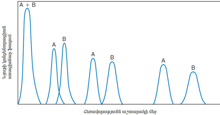
Նկար 8. Երկու A և B նյութերի բաշխումը քրոմատոգրաֆիական աշտարակում տիպական քրոմատոգրաֆիական բաժանման դեպքում
