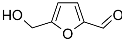
Նկար 5. 5-հիդրօքսիմեթիլֆուրֆուրոլի կառուցվածքային բանաձևը
