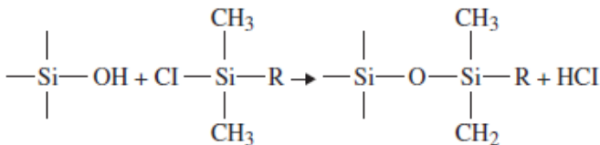
Նկար 12. Սիլիկագելի և մոնոքլորսիլանի միջև ռեակցիայի հավասարումը
