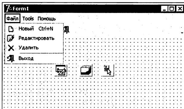
Рис. 11.46. Меню Файл
