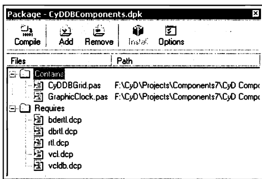
Рис. 19.2. Окно пакета
