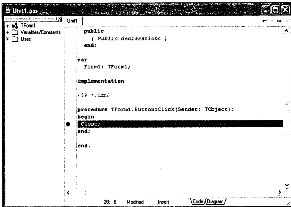
Рис. 24.1. Точка прерывания
