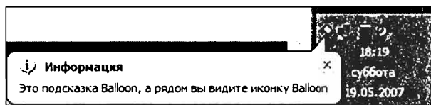
Рис. 11.52. Подсказка Balloon
