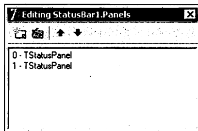
Рис. 11.39. Редактор панелей
