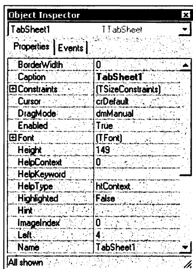
Рис. 11.29. Свойства страницы
