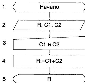
Рис. 2.2. Блок-схема сложения двух чисел
