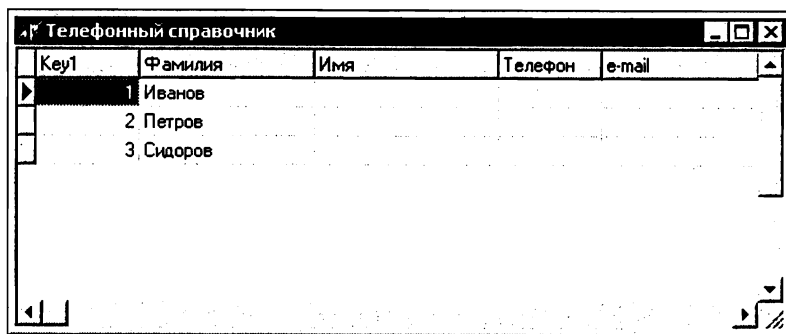
Рис. 14.7. Форма приложения
