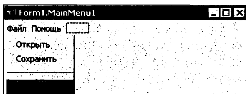
Рис. 9.6. Пример разделителя
