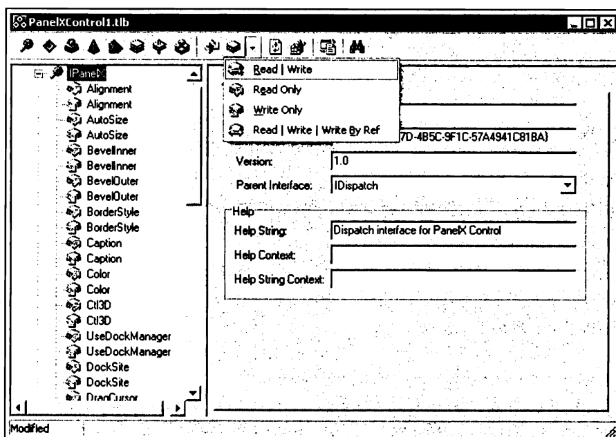
Рис. 21.11. Создание свойства
