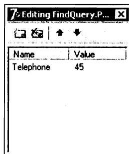
Рис. 14.26. Редактор параметров
