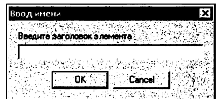
Рис. 11.35. Окно ввода
