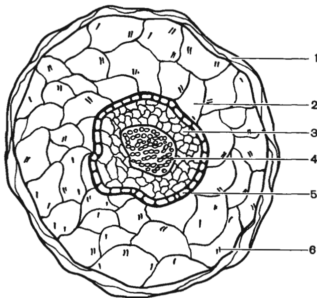
Рис. 171. Схема строения клубенька вейника лесного: 1 — кора; 2 — коровая паренхима; 3 — перициклическая паренхима; 4 — сосудистый пучок; 5 — эндодерма; 6 — бактерии (по И. Л. Клевенской).
