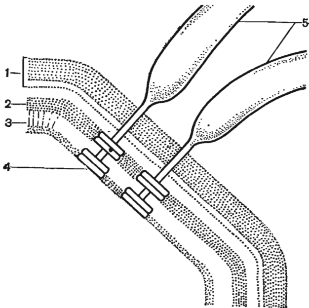
Рис. 18. Схема прикрепления жгутика:
