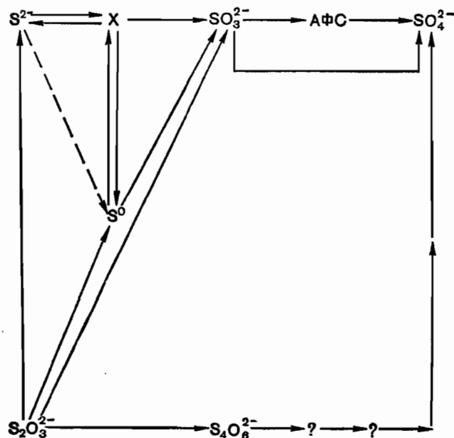
Рис. 139. Путь окисления соединений серы тионовыми бактериями.
