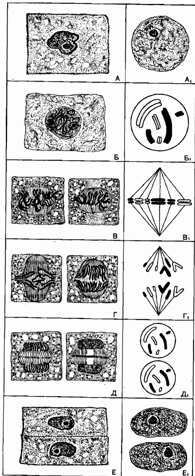
Рис. 37. Митотическое деление клетки кончика корешка лука (слева) и параллельно — схема деления материала ядра при митозе (справа). На схеме одна из гомологичных хромосом зачернена, другая изображена светлой.
