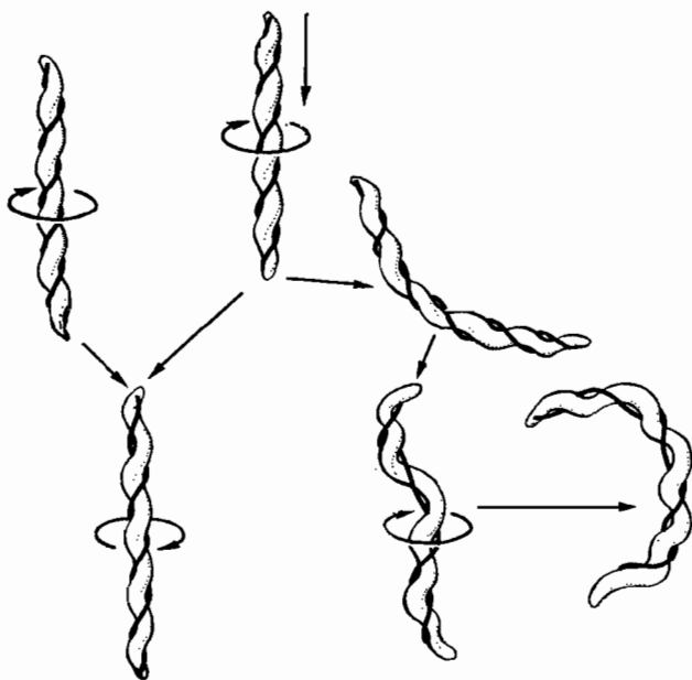
Рис. 116. Схема механизма движения спирохет.
