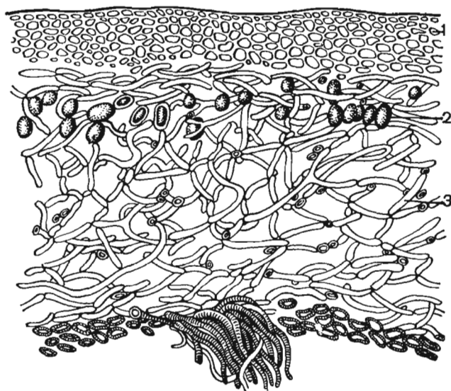
Рис. 8. Поперечный разрез лишайника: 1 — корковый слой; 2 — включения клеток водорослей; 3 — гифы гриба. Внизу видны ризоиды.
