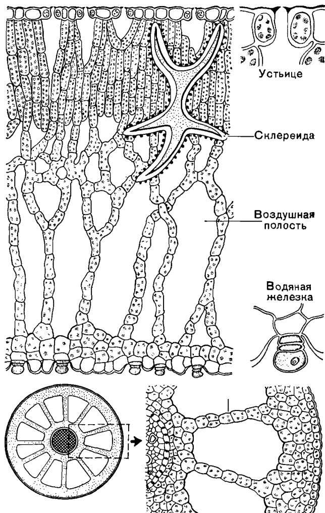
Рис. 49. Анатомическое строение некоторых водных растений. В в е р х у — поперечный разрез через плавающий лист желтой кувшинки; видны обширные воздушные полости; отдельно изображены устьице и водяная железка. В н и з у — поперечный разрез стебля урути, с п р а в а — при большом увеличении.
