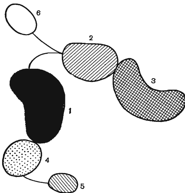
Рис. 77. Последовательность роста гиф и почек Pedomicrobium . (Цифры означают поэтапность перехода к росту разных участков гиф и почек.) Схема.
