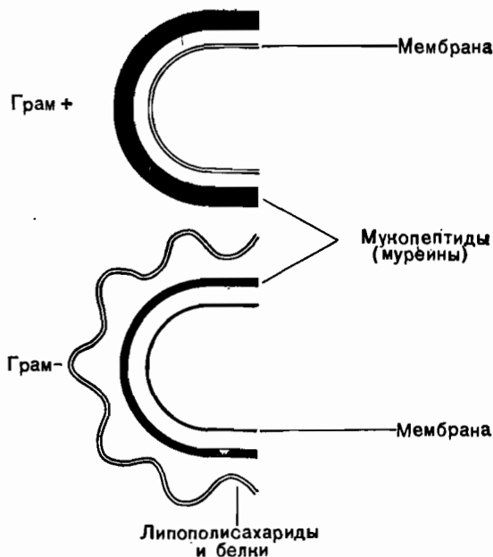
Рис. 21. Схема строения клеточных стенок грамположительных (Грамм +) и грамотрицательных (Грамм -) бактерий.
