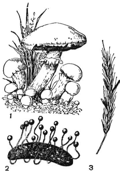
Рис. 6. Строение гриба: 1 — внешний вид гриба (шампиньон); 2 — прорастающий «плодом» спорыньи; 3 — спорынья на ржи.
