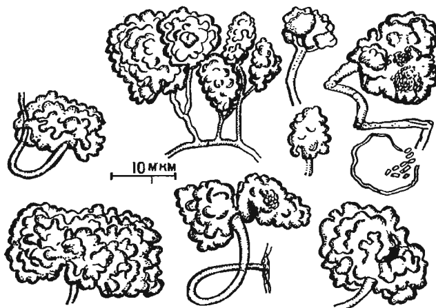
Рис. 93. Разнообразные формы спорангиев у Amorphosporangium .
