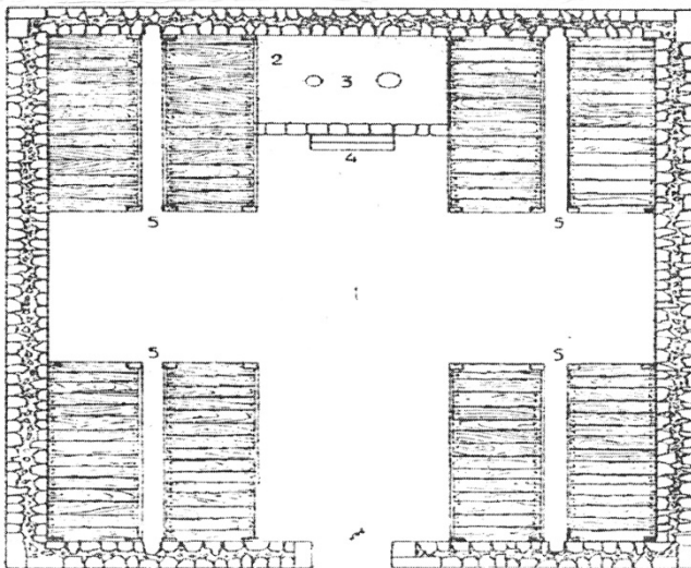
Թոնրատուն-գլխատուն, հատակագիծ, վերին (փոքր) և ցածի (մեծ) տուն, օդաներով
