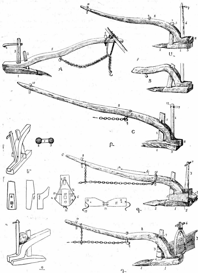
ա) Բարձր Հայքի արորներ (Ա, Բ), ճղլա (Գ), անձար գութան (Դ)
