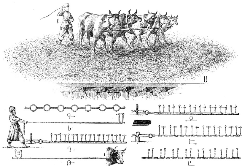
Կոռիով կալսելու եղանակ
