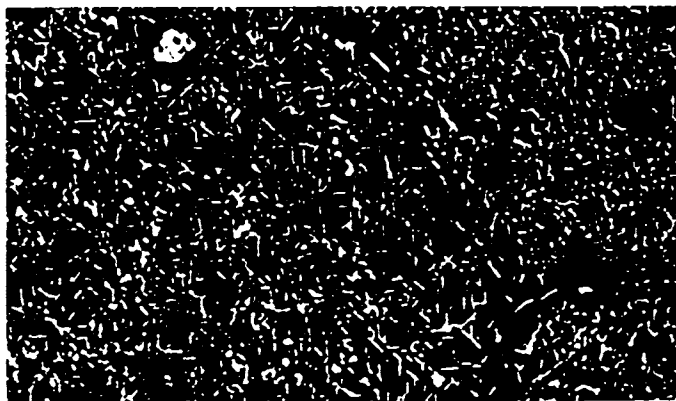
Метастабильные частицы в сплаве ВД23. Увеличено в 40 000 раз
