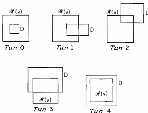
Рис. 2.29. Примеры различных типов пересечений D с R(v) , когда D \cap R(v) \neq \emptyset .
