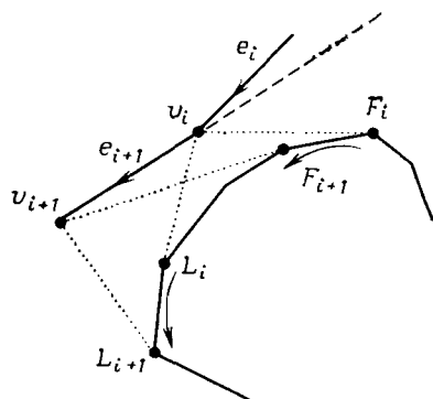
Рис. 7.29. Действия на общем шаге, если v_i — вогнутая вершина, а F_i лежит слева от луча \Lambda e_{i+1}v_{i+1} .
