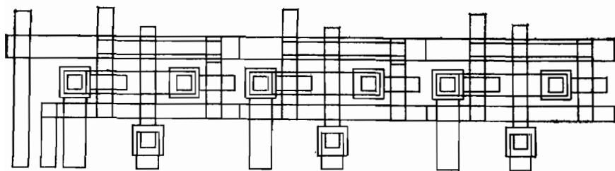
Рис. 8.1. Типичная геометрия одной интегральной схемы.
