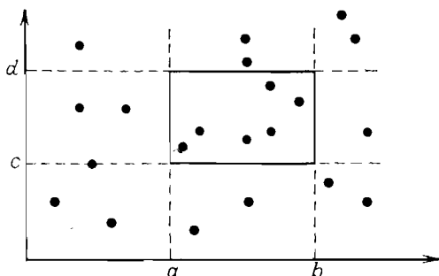
Рис. 2.1. Региональный запрос. Сколько точек внутри прямоугольника?.
