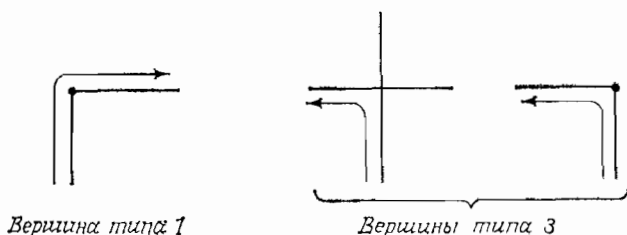
Рис. 8.26. Типы вершин.
