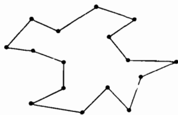
Рис. 6.3. Маршрут коммивояжера.
