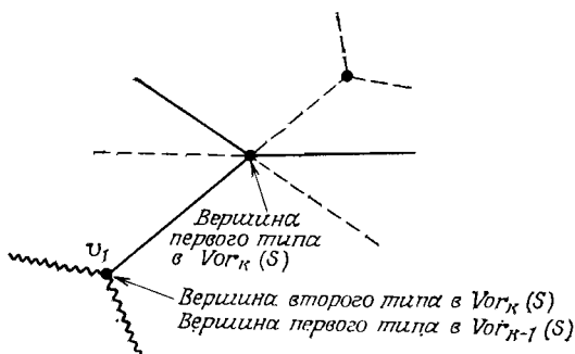
Рис. 6.16. Иллюстрация «жизненного цикла» вершины диаграммы Вороного.
