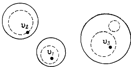
Рис. 1.10. Построение U_\varepsilon по U ; U ограничено сплошными линиями, U_\varepsilon — штриховыми.
