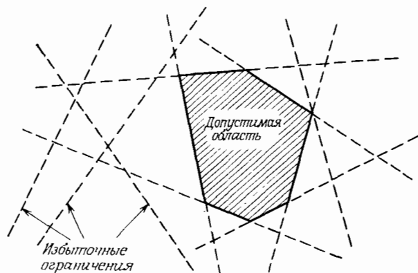
Рис. 7.17. Допустимая область множества линейных ограничений.
