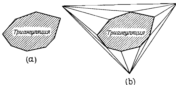
Рис. 2.18. Заданная триангуляция (а) и та же триангуляция внутри охватывающего ее треугольника (b).
