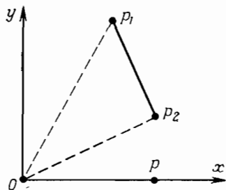
Рис. 3.5. Сравнение полярных углов путем вычисления ориентированной площади треугольника (O, p_2, p_1) .
