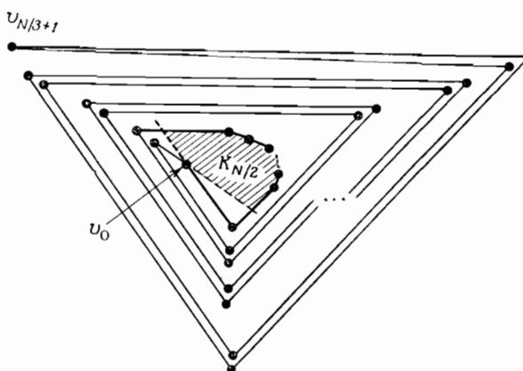
Рис. 7.32. Случай, когда немодифицированный алгоритм затрачивает O(N^2) времени. N -сторонний многоугольник K_{N/2} заштрихован. Затем алгоритм делает вокруг K_{N/2} N/12 оборотов, прежде чем достигает вершины V_{N/3+1} , в которой выясняется, что K(P) = \emptyset .
