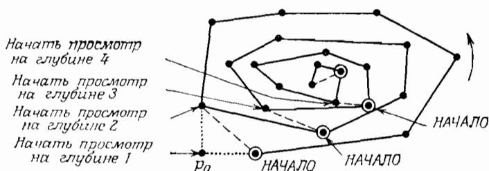
Рис. 4.14. Определение глубины точек множества путем многократного обхода по методу Джарвиса. Вершины, помечаемые последовательно меткой НАЧАЛО, обведены кружком.
