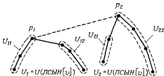
Рис. 3.20. Для построения В-оболочки объединения оболочек U_1 и U_2 необходимо построить общий опорный отрезок (мост) p_1 p_2 .
