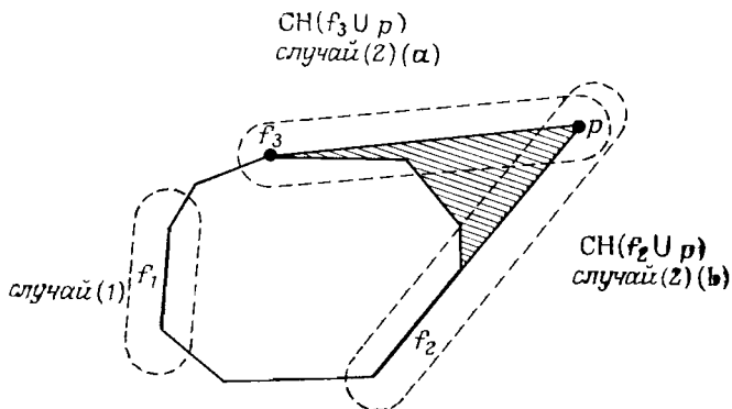
Рис. 3.27. Иллюстрация случаев, рассматриваемых в теореме 3.15.
