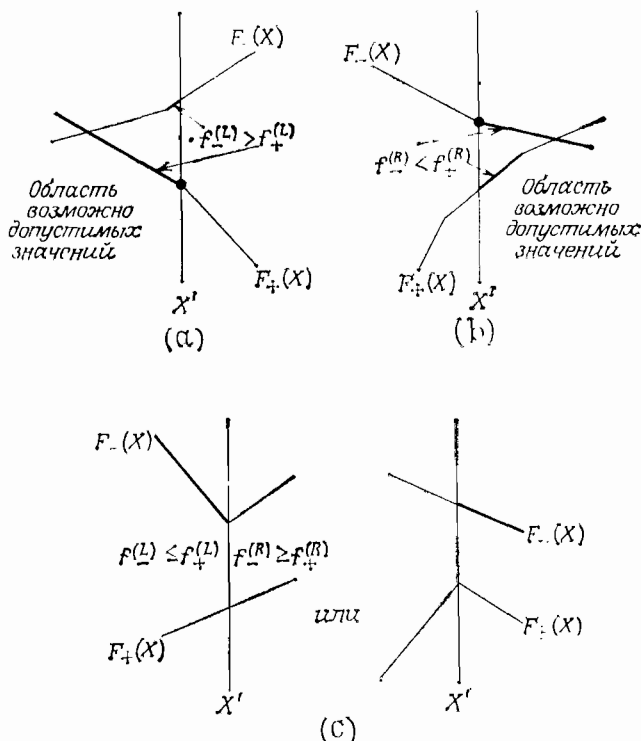
Рис. 7.22. Иллюстрация возможных случаев, при которых F_-(X) > F_+(X) .
