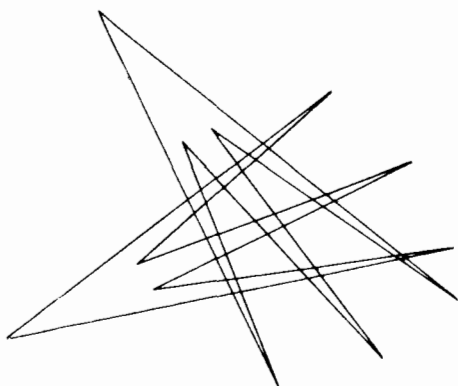
Рис. 7.11. Пересечение двух звездных многоугольников.
