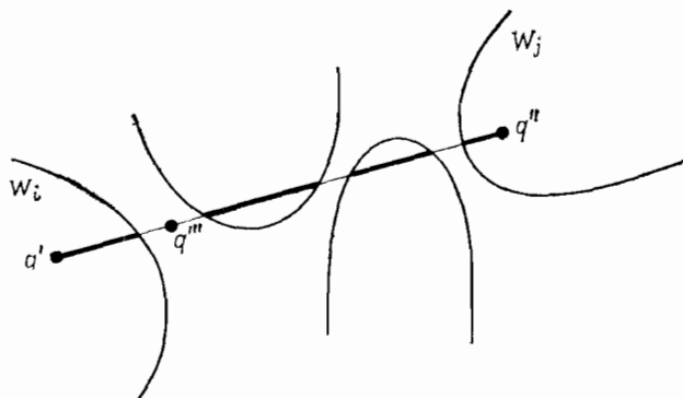
Рис. 1.9. Иллюстрация к доказательству того, что W_i = W_j .
