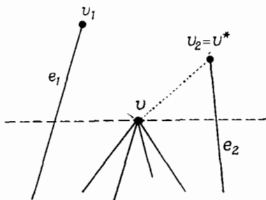
Рис. 2.14. Пример типичной нерегулярной вершины v .
