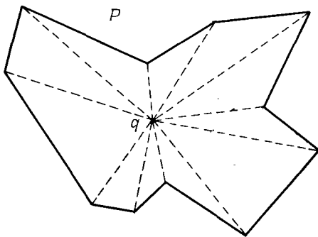
Рис. 2.7. Звездный многоугольник.
