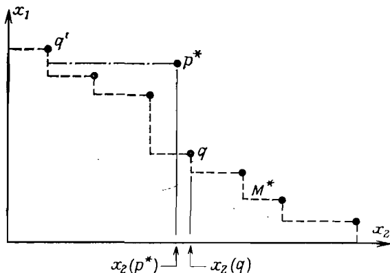
Рис. 4.4. Множество максимумов M^* можно линейно упорядочить. При этом проверка условия « p^* < M^* ?» заключается в сравнении x_1 -координаты точки p^* с x_1 -координатой ближайшей к p^* точки множества M^* , расположенной справа от нее.
