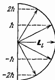
d -состояние
