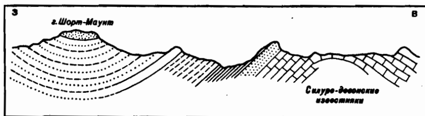
Схематический поперечный разрез Аппалачей
