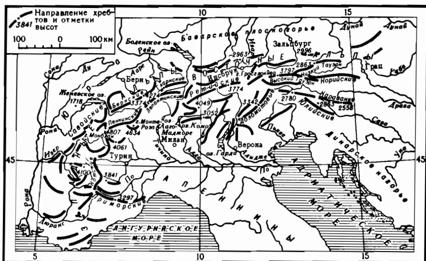
Орографическая схема Альп
