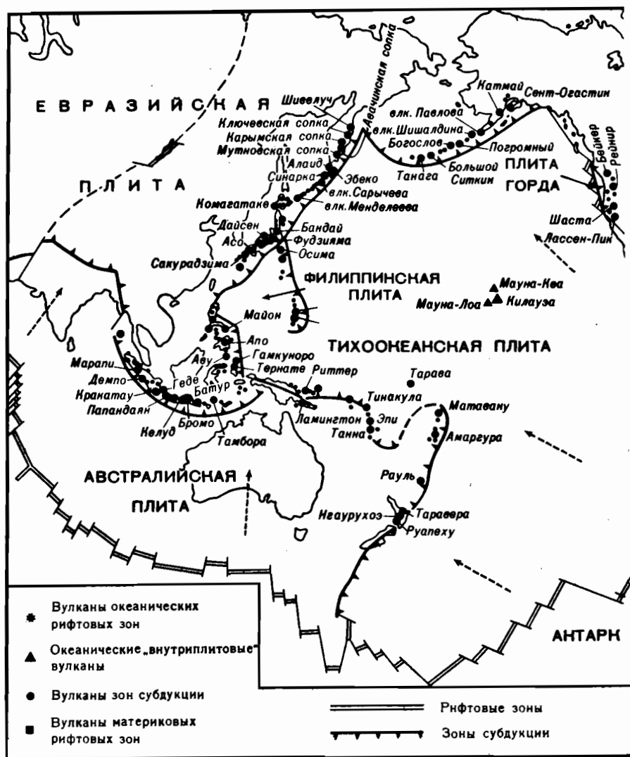
Литосферные плиты Земли. Вулканы (по Х. Расту)
