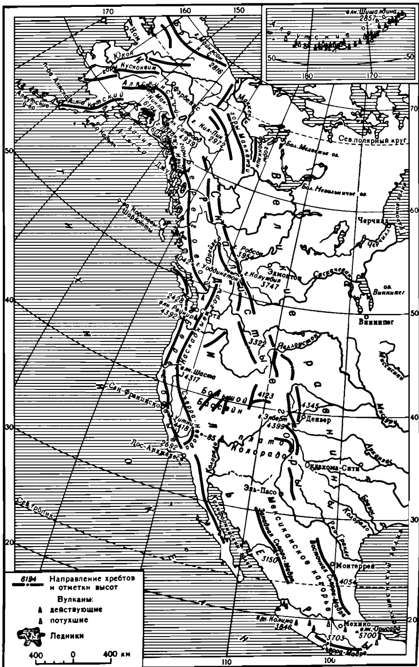
Орографическая схема Кордильер
