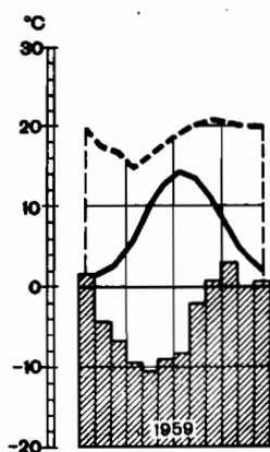
БЕРГЕН (Норвегия) выс. 43 м
