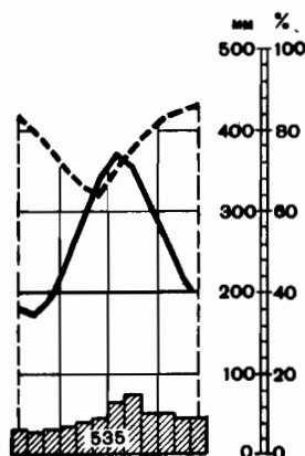
СТОКГОЛЬМ (Швеция) выс. 44 м
