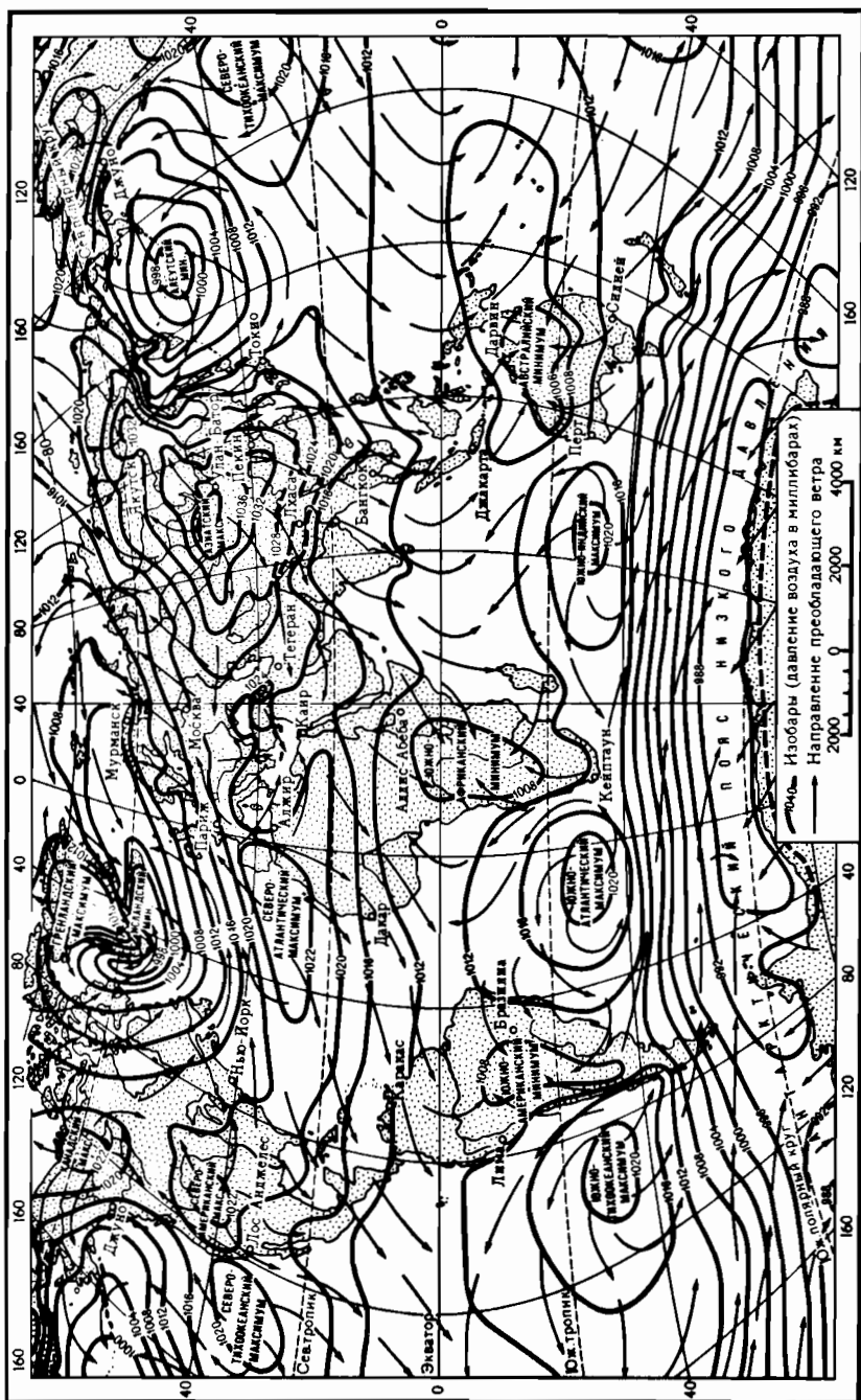
Давление воздуха и ветры в январе
