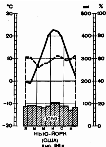
Годовой ход температур, осадков и относительной влажности на востоке США
