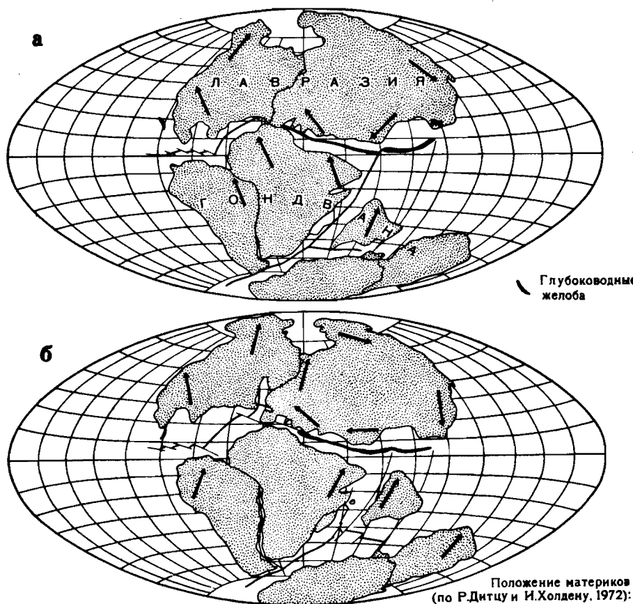
Схема раскрытия Тетиса
