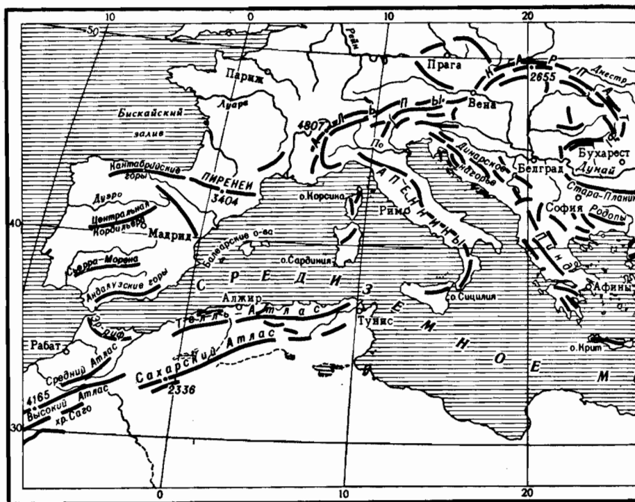
Орографическая схема Средиземноморья и Переднеазиатских нагорий
