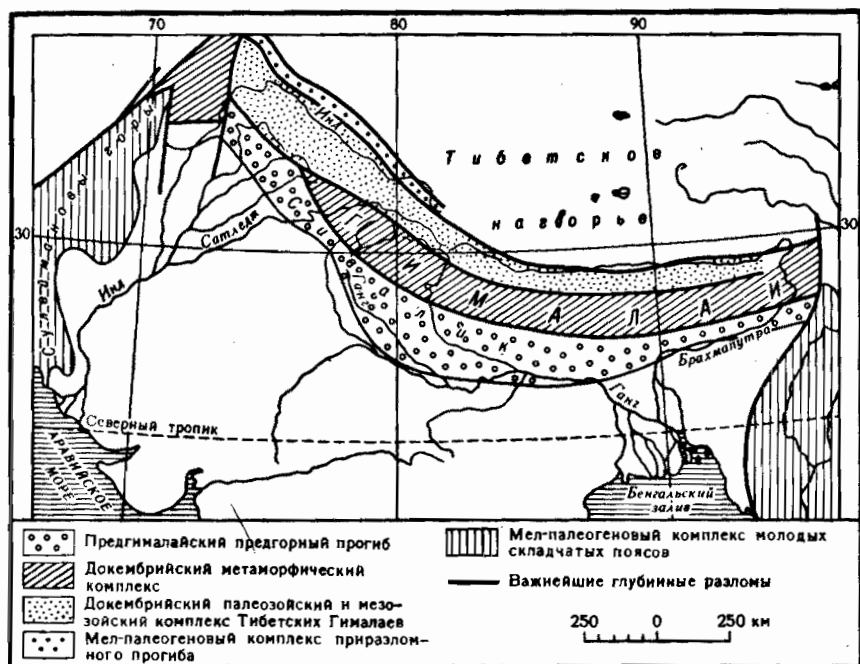
Тектоническая схема Гималаев
