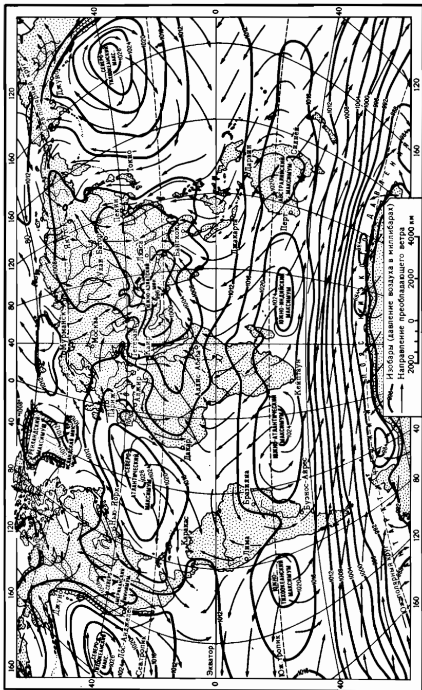
Давление воздуха и ветры в июле
