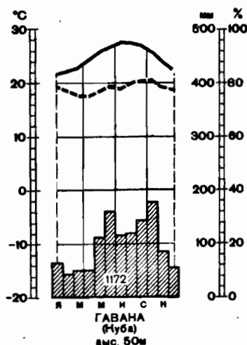
Годовой ход температур, осадков и относительной влажности на Кубе.
