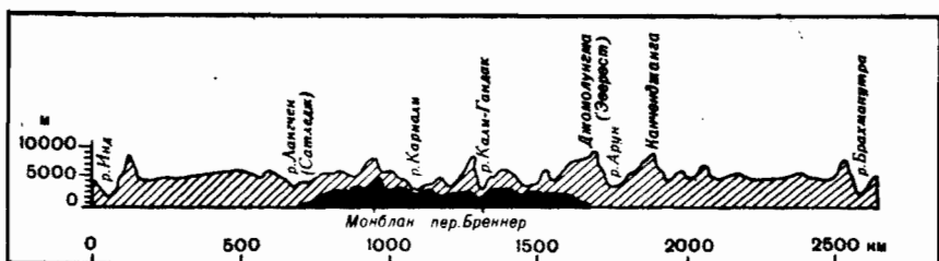
Сравнительный профиль Альп и Гималаев
