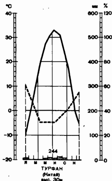
Годовой ход температур, осадков и относительной влажности в Турфанской котловине
