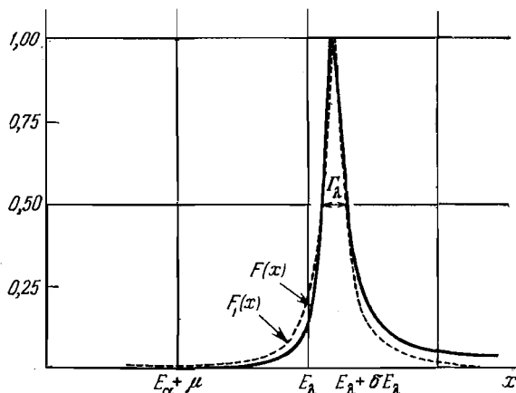
Рис. 27. Характерный вид функций F(x) и F_l(x) . Функции \Delta и \Gamma имеют энергетическую зависимость, типичную для дипольных переходов:
