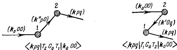
Рис. 20. Диаграммы амплитуд двойного рассеяния.
