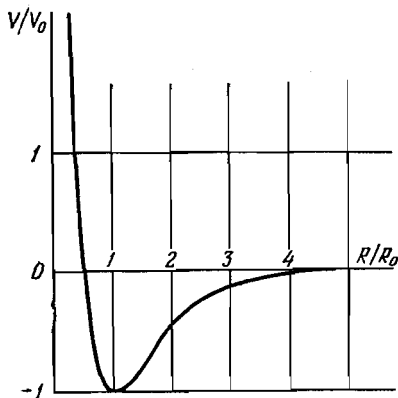
Рис. 15. Потенциал Морса V = V_0 (e^{-2(R-R_0)/b} - 2e^{-(R-R_0)/b}) . R_0 — расстояние между ядрами в положении равновесия, V_0 — значение потенциала в этой точке. Ширина минимума тем меньше, чем меньше отношение b/R_0 . На рисунке b/R_0 = 0,68 , что соответствует молекуле водорода.
