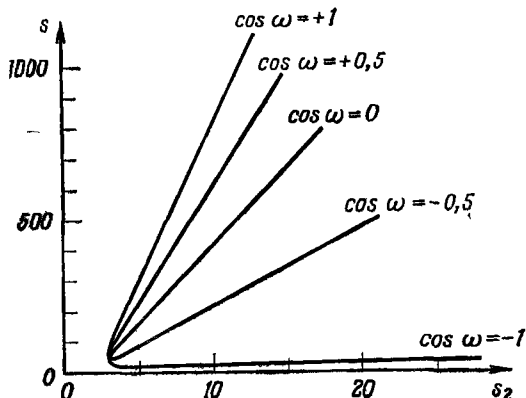
Фиг. 56. Кривые постоянных значений толлерева угла \omega на плоскости ss_2 . Прочие инварианты взяты равными s_1=8 , t_1=-4 , t_2=-5 ; выбрана реакция pp \rightarrow p\pi\Delta .
