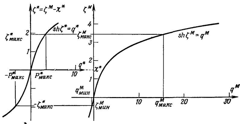
Фиг. 90. Соотношение q/m'_c = \operatorname{sh} \zeta в СЦМ и в системе мишени.
