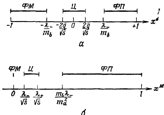
Фиг. 95. Области ФМ, ФП и Ц при конечных, но больших s в масштабах переменных x^* и x^M .
