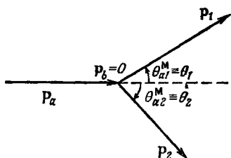
Фиг. 19. Углы рассеяния \theta_1 и \theta_2 в системе мишени; в этом случае \theta_1 и \theta_2 связаны между собой сложным образом.
