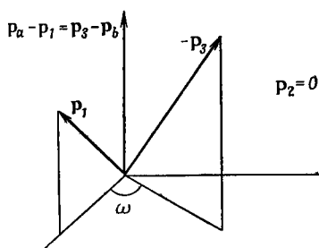
Фиг. 54. Геометрическое определение толлерова угла \omega в системе отсчета, в которой p_2 = 0 .
