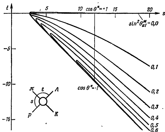
Фиг. 24. Физическая область для реакции \pi r \rightarrow \Lambda K в плоскости st .
