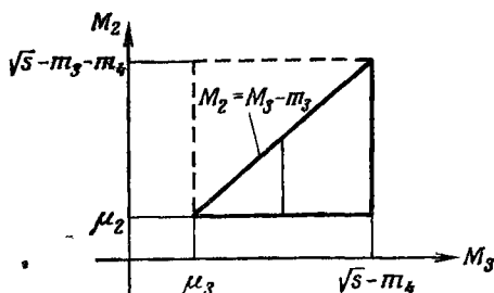
Фиг. 107. Область интегрирования по массам M_3 и M_2 при n=4 .
