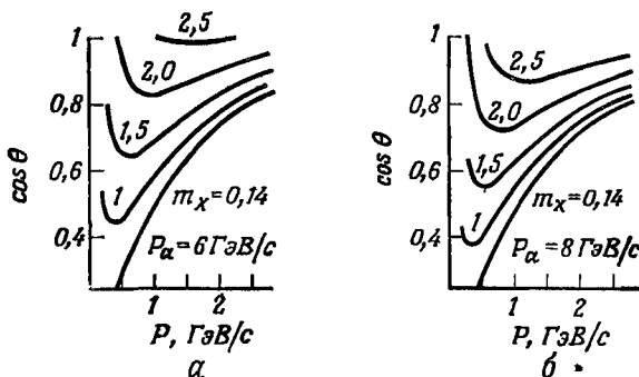
Фиг. 97. Зависимость \cos \theta от P при нескольких значениях недостающей массы m_X .
