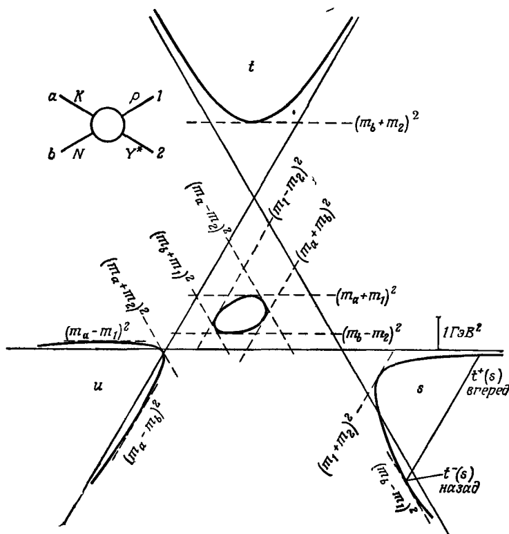
Фиг. 28. Физические области для реакции KN \rightarrow pY^* .
