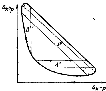
Фиг. 103. Диаграмма Далица для реакции \pi p \rightarrow \pi\bar{p} с перекрывающимися резонансными полосами.
