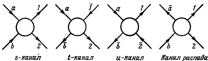
Фиг. 22. Различные каналы реакции p_a + p_b \rightarrow p_1 + p_2 и канал распада, который является физическим, если m_b > m_1 + m_2 + m_a .
