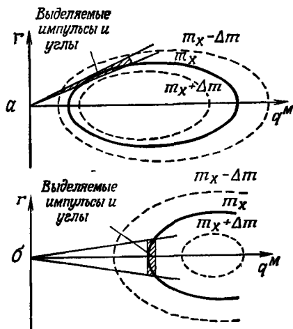
Фиг. 96. Область предельного угла (а) и область нулевого угла (б) в эксперименте по измерению недостающих масс в реакции a + b \rightarrow c + X ( q^M и r — составляющие импульса p , измераемого в системе мишени).
