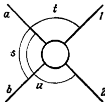
Фиг. 21. Инвариантные переменные для процесса p_a + p_b \rightarrow p_1 + p_2 .
