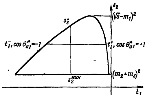
Фиг. 41. Диаграмма Чу—Лоу.
