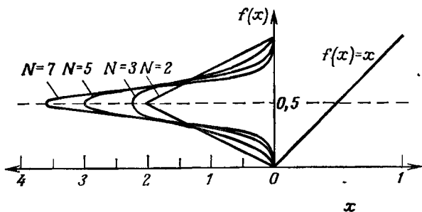
Фиг. 106. Иллюстрация сходимости интегрирования методом Монте-Карло.
