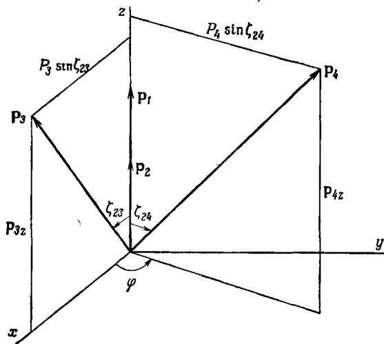
Фиг. 8. Псевдосферические координаты для p_4 в системе координат S(p_1, p_2, p_3) . 4-вектор p_1 пространственноподобен, его 0-компонента в этой системе равна нулю. Переменные P_i определяются равенством P_i^2 = p_{iz}^2 + p_i^2 .
