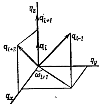
Фиг. 70. Векторы (3.13) в подпространстве xyz .
