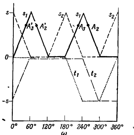
Фиг. 77. Зависимость s_1 , s_2 , t_1 , t_2 от \omega при m'_i = 0 . (Линейная форма зависимости — всего лишь приближение.)
