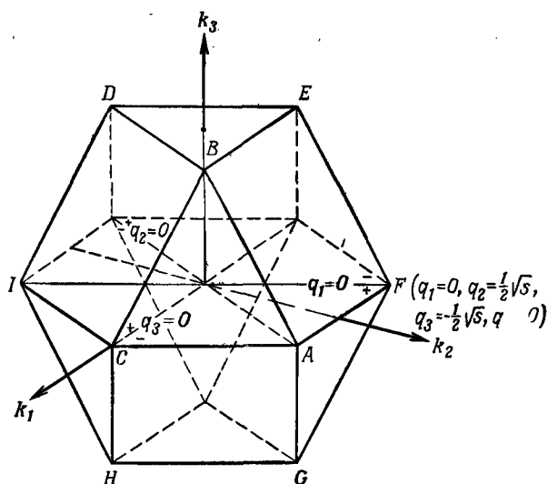
Фиг. 79. Система координат для случая q_1 + q_2 + q_3 + q_4 = 0 .
