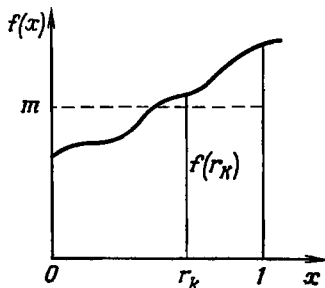
Фиг. 105. Интегрирование методом Монте-Карло функции f(x) на интервале (0, 1) ( r_k — случайная точка, m — точное значение интеграла).
