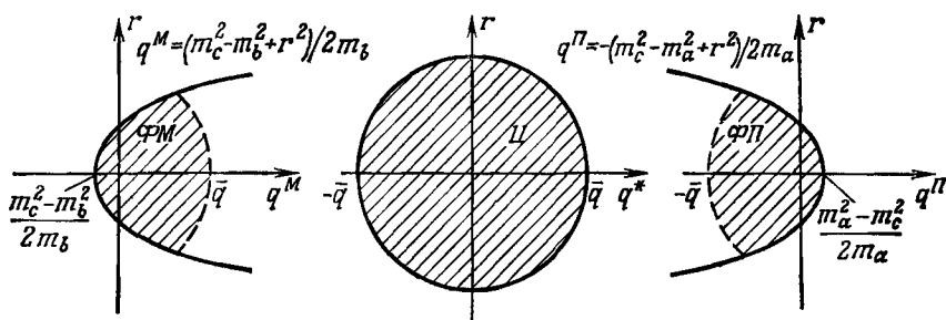
Фиг. 93. Области фрагментации мишени (ФМ) и падающей частицы (ФП) и центральная область (Ц) при s \rightarrow \infty ( \tilde{q} — некоторая конечная величина)
