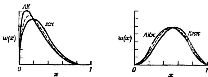
Фиг. 72. Распределение инвариантных масс пар АК, \pi\pi и троек АК \pi , К \pi\pi из реакции \pi^-p \rightarrow AK3\pi при 7 ГэВ/с в сравнении с его аппроксимацией (4.6) (штриховая линия).
