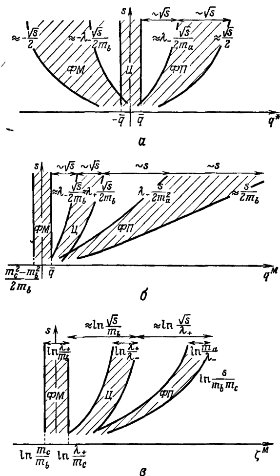
Фиг. 94. Качественное поведение интервалов (5.8), т. е. областей ФМ, ФП и U (фиг. 93) при s \rightarrow \infty ; а — в СЦМ, б — в системе мишени, в — на оси быстрот \zeta^M .
