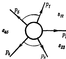
Фиг. 49. Аргументы у \Delta_4 можно выбрать таким образом, чтобы в определителе \Delta_4 = \Delta_4(p_5 + p_1, p_b, p_4, p_3 + p_4) инварианты s_{12} , s_{23} и s_{45} располагались симметрично.
