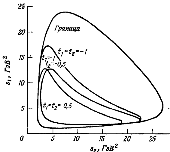
Фиг. 102. Кривая \Delta_4 = 0 для реакции pp \rightarrow p\pi\Lambda при 19 ГэВ/с, построенная при фиксированных значениях t_1 и t_2 , указанных на фигуре.
