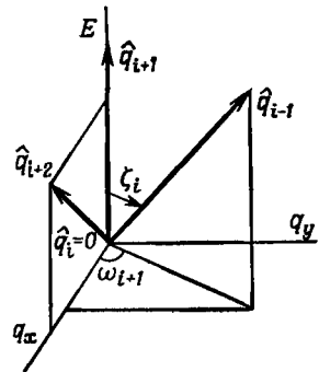
Фиг. 69. Расположение осей координат в системе отсчета S(q_i) , определяемой условием q_i = (0, 0, 0, \sqrt{-t_i}) .
