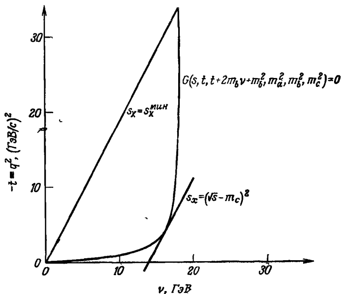
Фиг. 88. Физическая область для реакции pp \rightarrow pX при 19 ГэВ/с, полученная переходом от фиг. 87 к плоскости vt .
