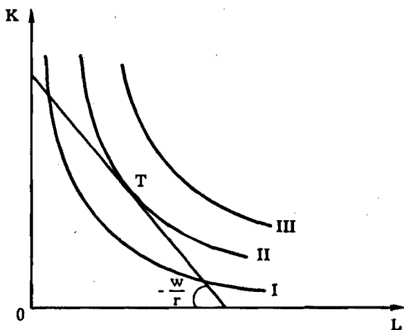
Рис. 5—7. Равновесие производителя
