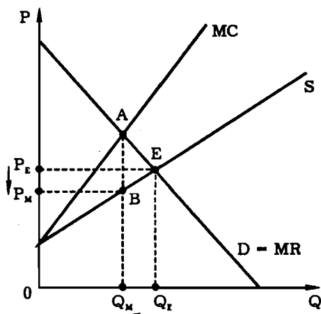
Рис. 8—12. Модель монополии
