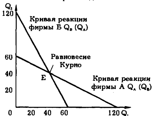
Рис. 8—3. Равновесие Курно
