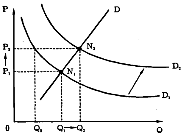
Рис. 4—16. Парадокс Гиффена
