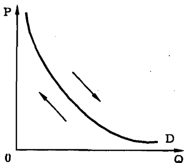
Рис. 3—3. Кривая спроса
