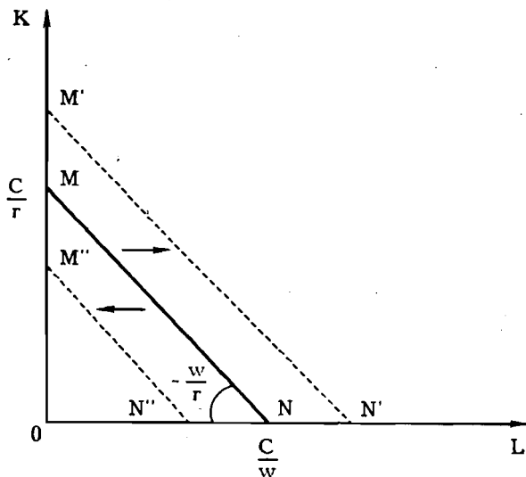
Рис. 5—6. Изокоста
