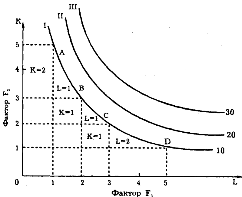
Рис. 5—4. Изокванты
