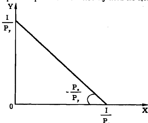
Рис. 4—10. Бюджетное ограничение
