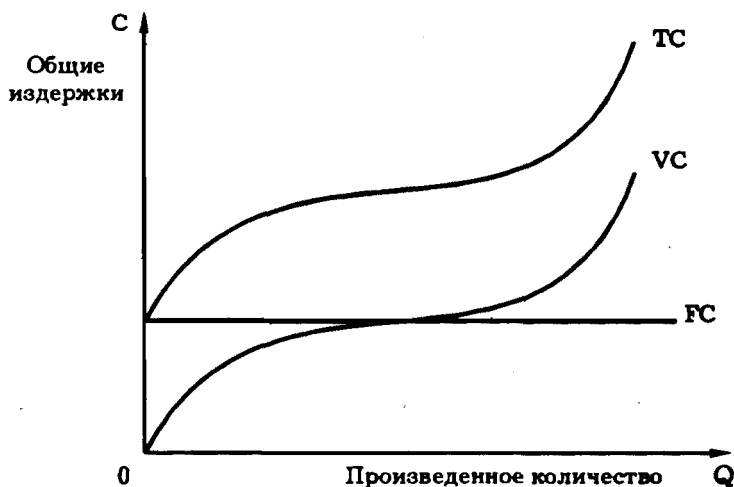
Рис. 6—11. Общие издержки
