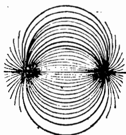
Рис. 76. Диполь
