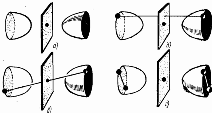
Рис. 59. а. q_1 = e — тождественное преобразование, б. q_2 — отражение в плоскости yz , в. q_3 — отражение в точке 0, г. q_4 — отражение в плоскости xy
