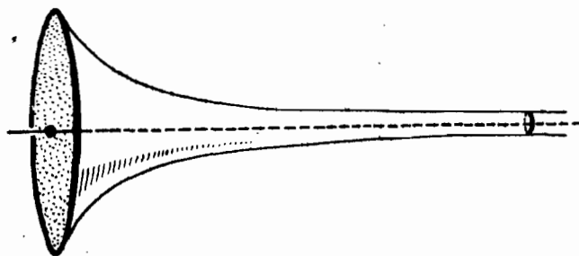
Рис. 23. Поверхность Бельтрами
