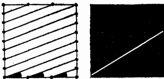
Рис. 29. Слева \operatorname{tg} \alpha — рациональное число, справа — иррациональное
