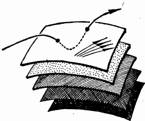
Рис. 64. Такой интегральной траекторией быть не может
