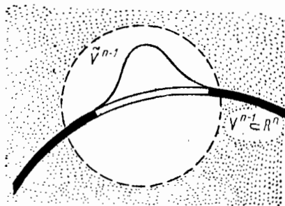
Рис. 35. Объем \tilde{V}^{n-1} \geq объем V^{n-1}
