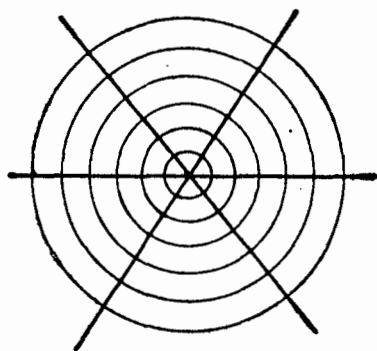
Рис. 74. Потенциал \Phi(x, y) — многозначная функция
