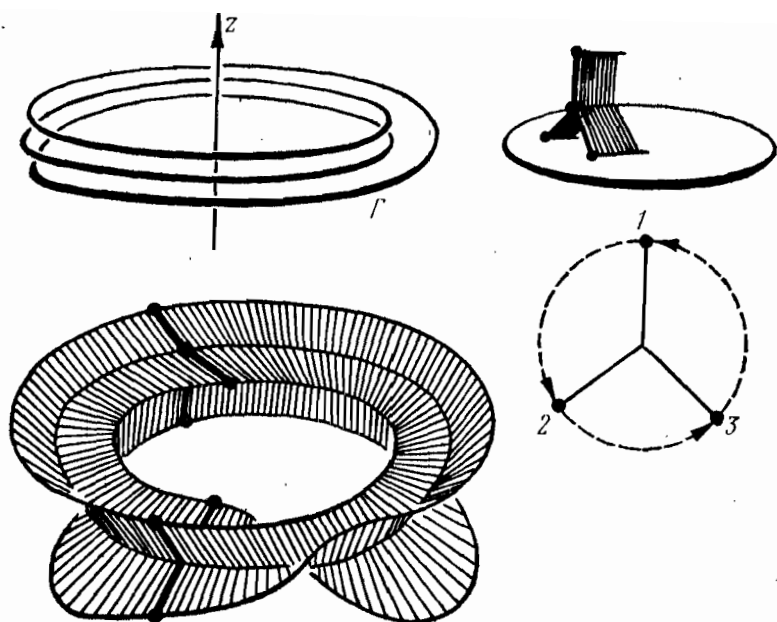
Рис. 44. \sigma = \begin{pmatrix} 123 \\ 231 \end{pmatrix}
