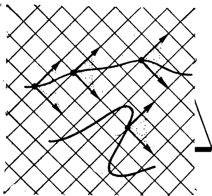
Рис. 17. Мировой линии, изображенной внизу, быть не может
