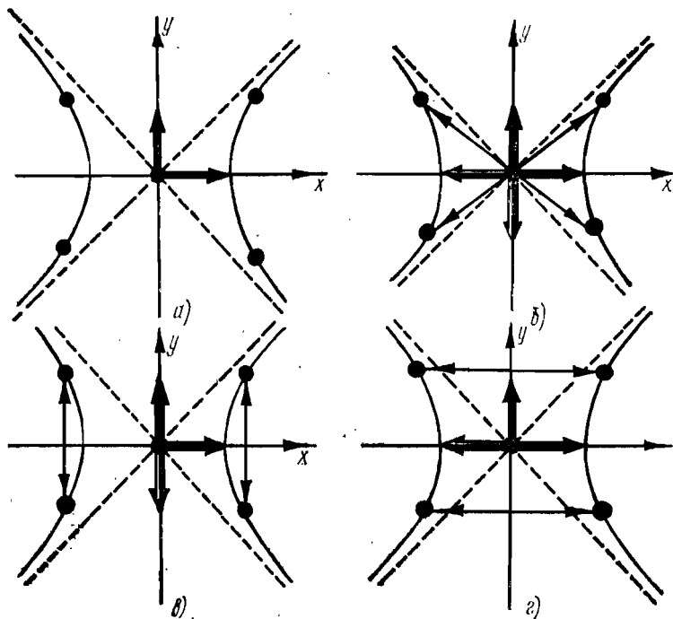
Рис. 53. а. g_1 = e = \begin{pmatrix} 1 & 0 \\ 0 & 1 \end{pmatrix} — тождественное преобразование
