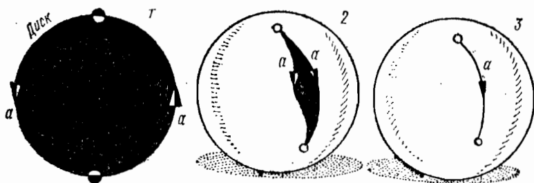
Рис. 112. W = aa^{-1} — не триангуляция
