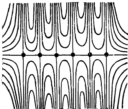
Рис. 78. k=6
