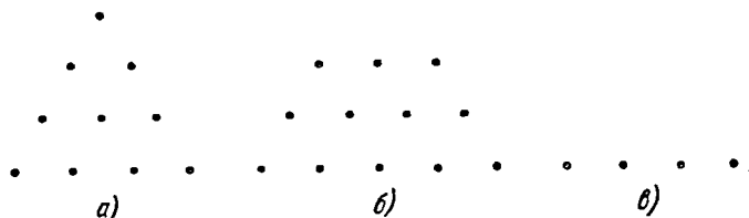
Рис. 52. Треугольные и трапецидальные числа.
