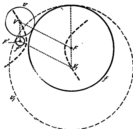
Рис. 59г. Что такое гипербола?
