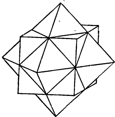
Рис. 60а. Глядя на K и O представьте себе P и Ob .
