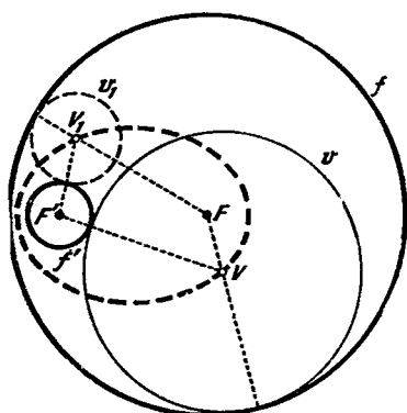
Рис. 59а Что такое эллипс?
