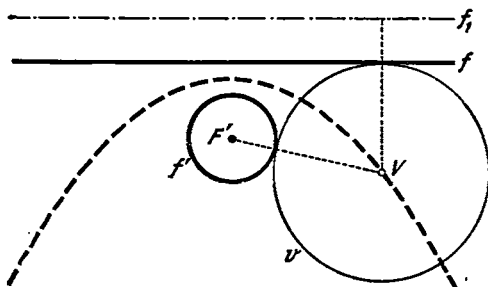
Рис. 59в. Предельный случай эллипса.
