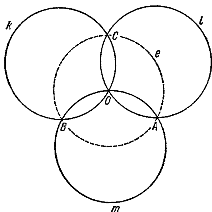
Рис. 40а. Три окружности, проходящие через одну точку.
