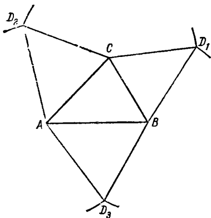
Рис. 45а. Постройте тетраэдр по шести его ребрам.
