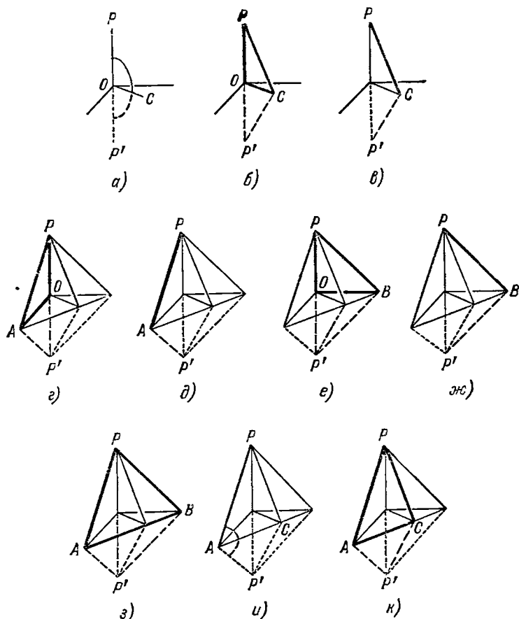
Рис. 34. Геометрическая фигура в переменном аспекте.
