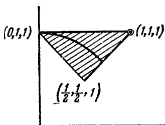
Рис. 47д. ... и для вырожденных треугольников.
