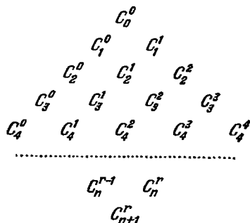
Рис. 16в. Символический треугольник Паскаля.
