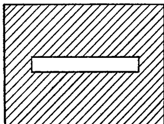
Рис. 11. С помощью двух разрезов — квадрат!
