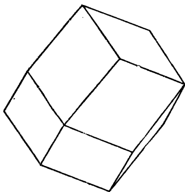
Рис. 60в. Выпуклая оболочка Ob .
