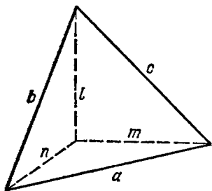
Рис. ба. Теорема Пифагора в пространстве.
