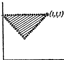
Рис. 47б. Проверка для равностороннего треугольника.
