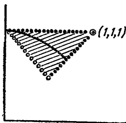
Рис. 47в. ...и для прямоугольных треугольников.
