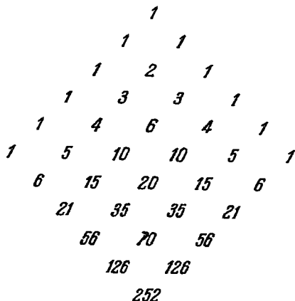
Рис. 166. Квадрат, вырезанный из треугольника.
