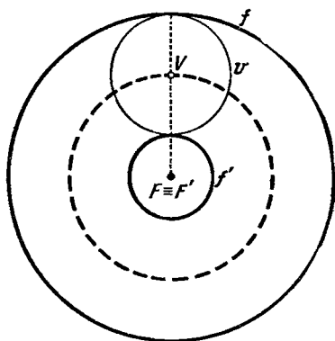
Рис. 59б Фокусы эллипса совпали.
