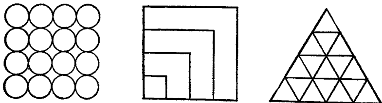
Рис. 18б. Четвертое квадратное число.
