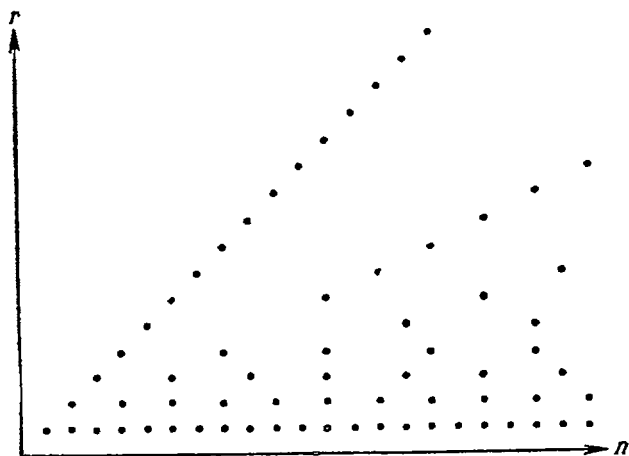
Рис. 53б. Для вдумчивого читателя (чертеж Лейбница): r является делителем n .
