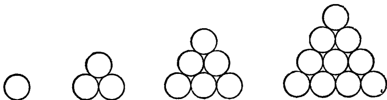
Рис. 18а. Первые четыре треугольных числа.
