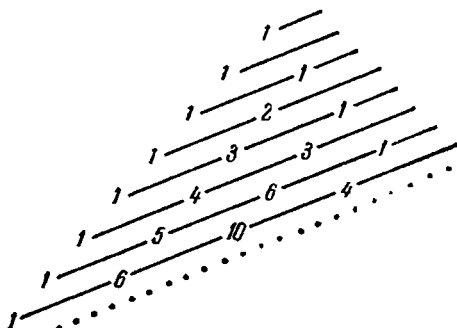
Рис. 19а. Истолкование чисел Фибоначчи с помощью наклонных линий.
