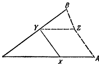
Рис. 1г. Связь с ранее уже известным.
