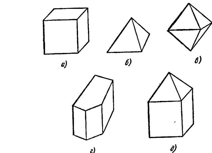
Рис. 49. Многогранники.
