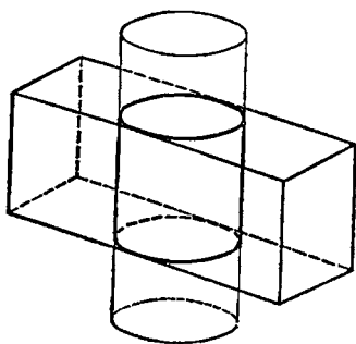
Рис. 27в. Два геометрических места.
