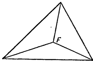
Рис. 45б. Один аспект задачи.
