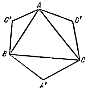
Рис. 37б. Больше связей.
