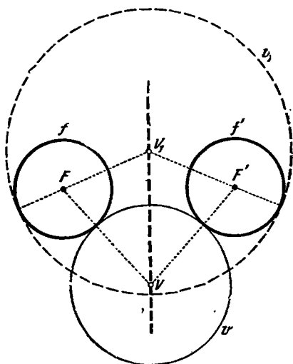
Рис. 59д. Частный случай гиперболы.
