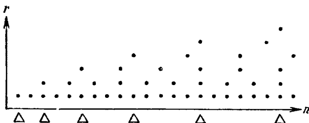
Рис. 53а. Трапецидальное представление числа n с помощью r рядов.
