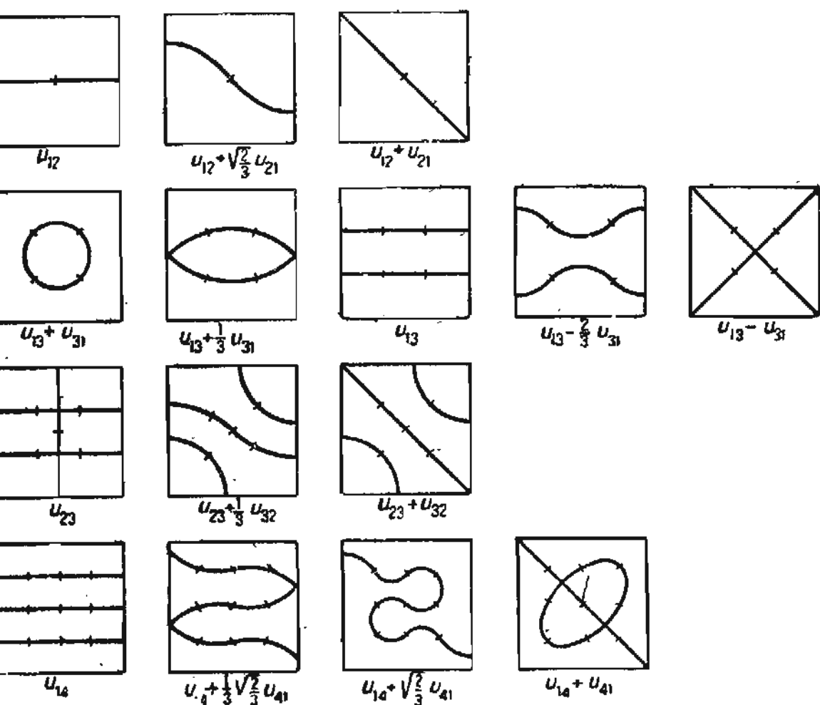
Черт. 2. Узловые линии квадратной мембраны.
