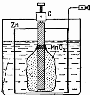
Рис. 122. Элемент Лекланше
