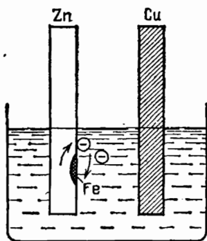
Рис. 120. Возникновение паразитных токов в гальваническом элементе
