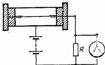
Рис. 157. Схема устройства счетчика Гейгера — Мюллера для элементарных частиц
