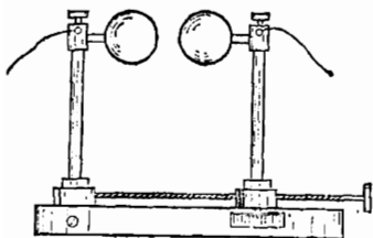
Рис. 152. Искровой вольтметр
