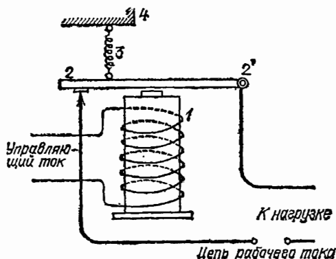
Рис. 370. Электромагнитное реле
