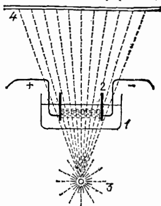
Рис. 25. Схема экспериментальной установки для получения картин электрического поля: 1 — кювета, содержащая касторовое масло с кристалликами хинина, 2 — проводники, соединенные с электрической машинной и создающие электрическое поле, 3 — источник света, 4 — экран, на который проецируется тень от кристалликов
