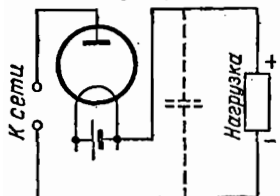
Рис. 315. Схема однополупериодного выпрямителя
