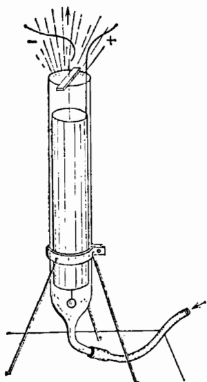
Рис. 156. Простейший вид электрофильтра
