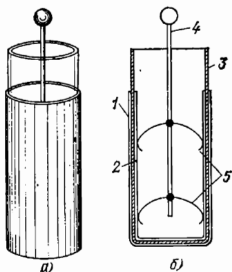
Рис. 59. Лейденская банка: а) общий вид; б) схема устройства, 1 и 2 — станиольевые обкладки, 3 — стеклянный стакан, 4 — металлический стержень, 5 — упругие металлические полоски для контакта
