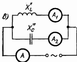
Рис. 302. Сопротивления в параллельных ветвях цепи переменного тока различны по своей природе
