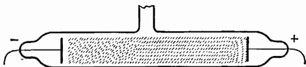
Рис. 162. Тлеющий разряд
