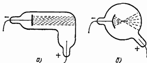
Рис. 169. Катодные лучи распространяются вдоль прямых линий, перпендикулярных к поверхности катода. Их направление не зависит от положения анода: а) плоский катод дает пучок параллельных лучей;
