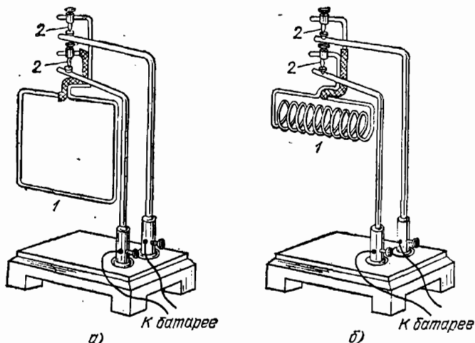
Рис. 203. Прибор Ампера для обнаружения действия магнитного поля Земли на виток с током: а) свободно подвешенный виток устанавливается так, чтобы плоскость его была перпендикулярна к меридиану; б) виток заменен катушкой
