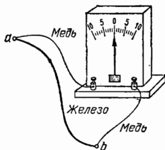
Рис. 114. В замкнутой цепи, составленной только из проводников первого рода, ток не возникает: а и б — спаи двух металлов
