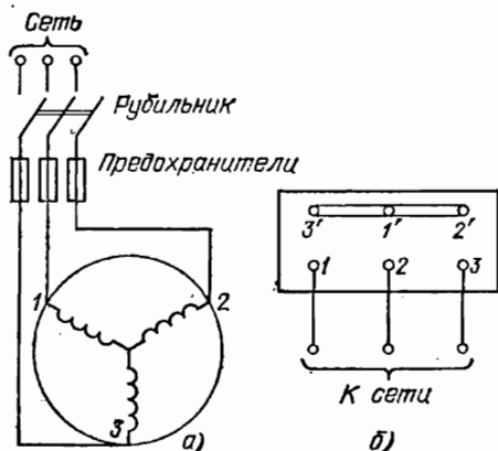
Рис. 355. Включение обмоток статора звездой: а) схема включения двигателя; б) соединение зажимов на щитке. Зажимы 1' , 2' , 3' соединены «накоротко» металлическими шинами; к зажимам 1 , 2 , 3 присоединены провода трехфазной сети
