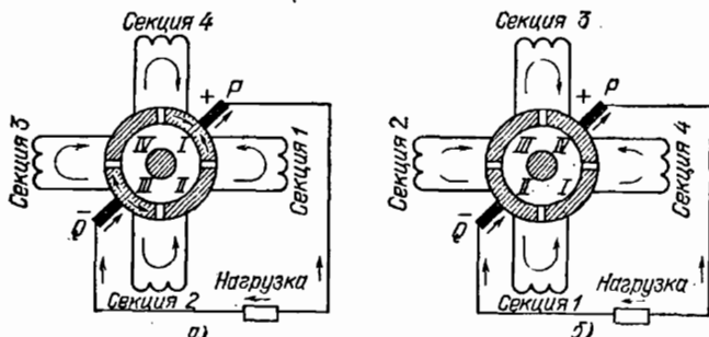
Рис. 336. Схема присоединения секций якоря к щеткам в два момента времени, отстоящие на четверть периода: a ) одна ветвь содержит секции 1 и 2, а другая — секции 3 и 4; б ) первая ветвь содержит секции 4 и 1, а вторая — секции 2 и 3. Во внешней цепи (нагрузке) ток всегда идет от P к Q
