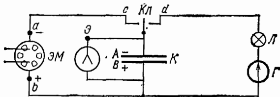
Рис. 70. Опыт для выяснения понятий о токе и э. д. с.: K — конденсатор, Л — лампочка карманного фонаря, Г — гальванометр, ЭМ — электрическая машина, Э — электрометр, Кл — ключ
