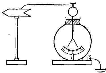
Рис. 45. Измерение разности потенциалов между проводником и Землей при помощи электрометра (первый способ)
