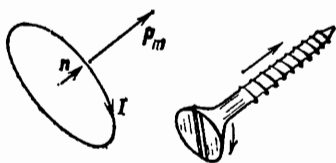
Рис. 211. Вращение головки винта в направлении тока I вызывает перемещение винта в направлении вектора \mathbf{n}
