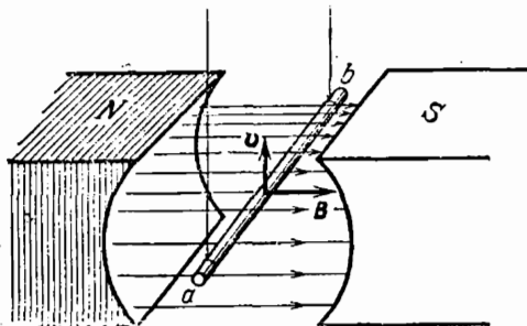
Рис. 268: К объяснению электромагнитной индукции при помощи силы Лоренца. Между точками a и b стержня индуцируется э. д. с., направленная от точки b к точке a
