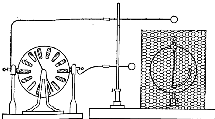
Рис. 53. Опыт Фарадея
