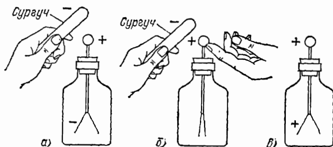
Рис. 16. Различные стадии зарядки тела через влияние: а) приближая к шарiku электроскопа отрицательно заряженный сургуч, мы вызываем на стержне электроскопа положительный заряд, а на его листках — отрицательный заряд; б) не убирая сургуча с отрицательным зарядом, прикасаемся рукой к шарiku электроскопа и отводим часть отрицательного заряда электроскопа через свое тело в землю; листки электроскопа спадают; в) убрав палец, а затем убрав сургуч, мы оставляем на электроскопе только положительный заряд, который распределяется между шариком и листками электроскопа
