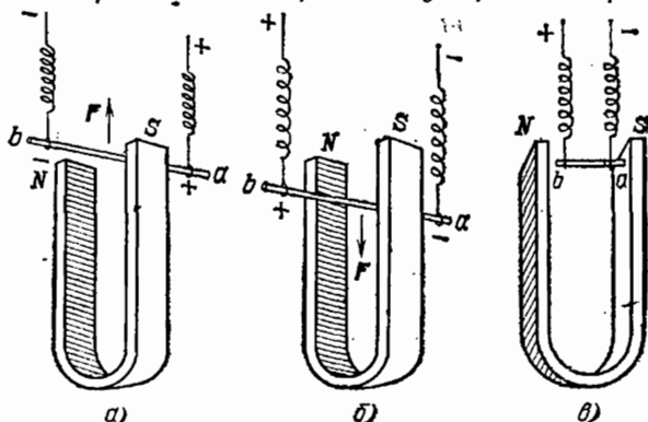
Рис. 234. При перемене направления тока изменяется направление силы F : проводник с током, который выталкивался из магнитного поля (а), начинает втягиваться в него (б). Если направление тока параллельно линиям магнитного поля, то оно не действует на проводник с током (в)
