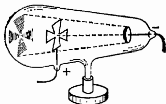
Рис. 165. Катодные лучи задерживаются металлической пластинкой, бросающая «тень» на стенку трубки
