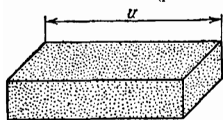
Рис. 183. К выводу соотношения \sigma = nuq
