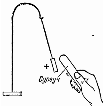
Рис. 7. Бумажная гильза, заряженная от стекла, притягивается к назлектризованному сургучу
