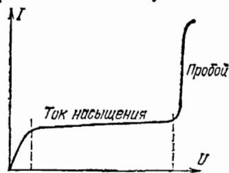
Рис. 150. Вольтамперная характеристика при переходе от несамоостоятельного разряда к самостоятельному
