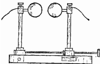
Рис. 152. Искровой вольтметр
