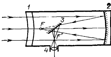
Рис. 259. Схема телескопа Максутова
