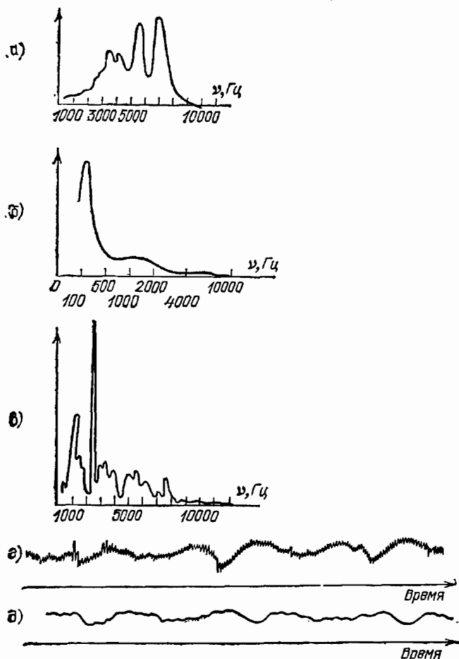
Рис. 45. Спектр шума согласной «с» (а), булзеновской горелки (б), пылесоса (в) и осциллограмма шума выхлопа мотора без глушителя (г) и с глушителем (д)
