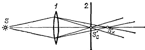
Рис. 235. Хроматическая aberrация: изображение точки S в синих лучах S'_с не совпадает с изображением в красных лучах S'_к . Рисунок имеет цветной дубликат (см. форзац)
