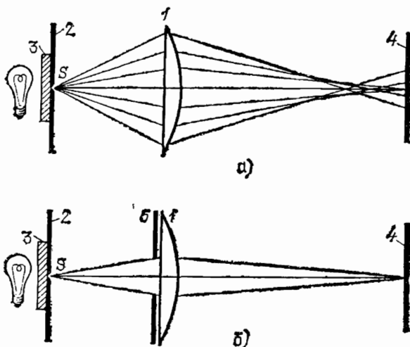
Рис. 228. Экспериментальное изучение сферической аберрации: а) линза, на которую падает широкий пучок, дает расплывчатое изображение; б) центральная зона линзы дает хорошее резкое изображение
