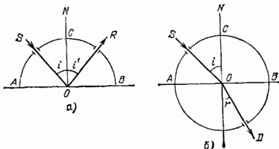
Рис. 181. Измерение угла отражения (а) и преломления (б)
