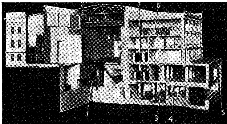
Рис. 410. Общий вид атомной электростанции (1954 г.): 1 — реактор, 2 — подъемный кран для замены «выгоревших» урановых стержней, 3, 4 — насос с электродвигателем, обеспечивающий циркуляцию воды через реактор, 5 — теплообменник, 6 — помещение управления реактором (пульт управления), 7 — щит с приборами, сигнализирующими о появлении недопустимой радиоактивности в различных помещениях станции
