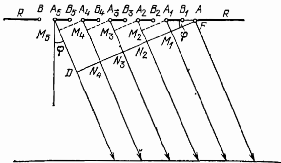
Рис. 281. К теории дифракционной решетки
