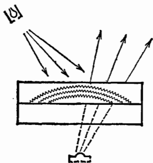
Рис. 289. Схема восстановления мнимого изображения
