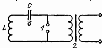
Рис. 51. Схема искрового возбуждения колебаний в контуре
