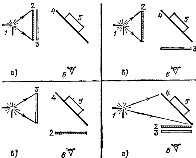
Рис. 347. К упражнению 40: 1 — дуга, 2 — фиолетовый фильтр, 3 — желто-зеленый фильтр, 4 — лист бумаги, 5 — сосуд с флюоресцином, 6 — глаз
