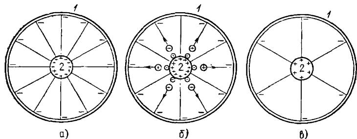
Рис. 385. К механизму работы газоразрядного счетчика частиц (1 — цилиндр счетчика, 2 — нить, диаметр которой преувеличен): а) Счетчик заряжен до рабочей разности потенциалов, при которой прохождение заряженной частицы через счетчик вызывает в нем вспышку газового разряда. Изображены линии электрического поля в счетчике. Густота линий, т. е. напряженность электрического поля, наибольшая у нити; б) поле в счетчике в момент самогашения разряда. Электроны, образованные при ионизации газа, собрались на нити и компенсируют часть ее положительного заряда. Положительные ионы продолжают двигаться к цилиндру. Поле у нити ослаблено; в) поле в счетчике, не присоединенном к батарее, после того как разряд погас и положительные ионы дошли до цилиндра.
