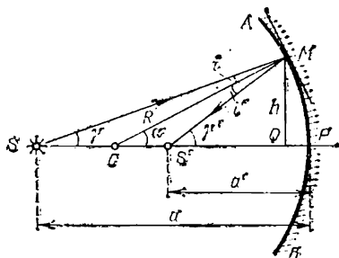
Рис. 205. Отражение от сферического зеркала луча SM , выходящего из точки S на оси
