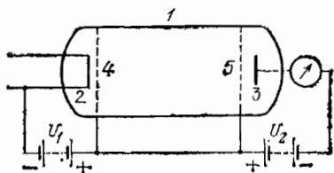
Рис. 359. Устройство для измерения потери энергии электроном при движении в парах ртути: 1 — стеклянная трубка, заполненная парами ртути (давление — тысячные доли мм рт. ст.), 2 — накаливаемый катод (нагреватель на чертеже не указан); 3 — анод, 4 и 5 — редкие металлические сетки, соединенные между собой, U_1 и U_2 ускоряющая и тормозящая разность потенциалов
