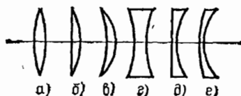
Рис. 198. Различные типы линз. Если материал линз преломляет сильнее, чем окружающая среда, то типы a , b , c — собирающие; типы d , e — рассеивающие
