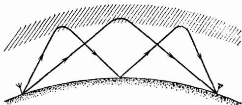
Рис. 149. Различные пути волны от передатчика к приемнику
