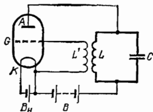
Рис. 58. Ламповый генератор
