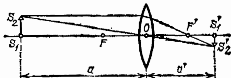
Рис. 211. Линейное увеличение линзы \beta = S'_1S'_2/S_1S_2 = a'/a
