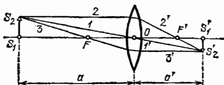
Рис. 215. Различные приемы построения изображения в линзе
