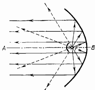
Рис. 161. Продольное сечение зеркала прожектора
