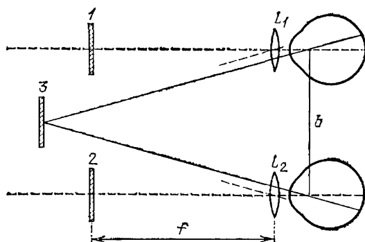
Рис. 262. Схема стереоскопа
