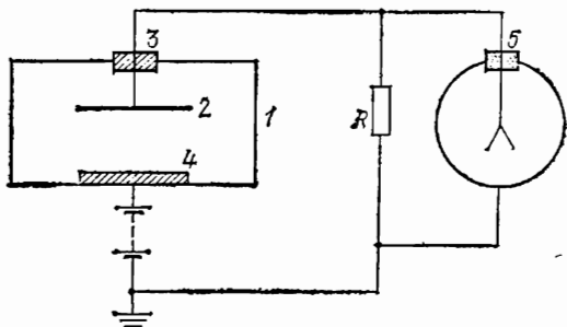
Рис. 376. Измерение ионизационного тока: 1 — корпус ионизационной камеры, 2 — электрод, отделенный от 1 изолирующей пробкой 3, 4 — изучаемый препарат, 5 — электрометр. Сопротивление R=10^9 - 10^{12} Ом. При достаточно высоком напряжении батареи все ионы, образуемые в объеме камеры ионизирующим излучением, собираются на электроды, и через камеру течет ток, пропорциональный ионизационному действию препарата. В отсутствие ионизирующих агентов воздух в камере является непроводником, и ток равен нулю
