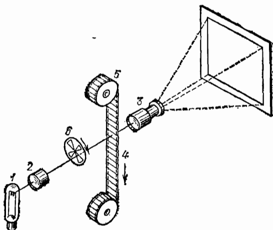
Рис. 241. Схема простейшего киноаппарата: 1 — источник света; 2 — конденсор; 3 — проекционный объектив; 4 — фильм; 5 — лентопритяжный механизм; 6 — obturator
