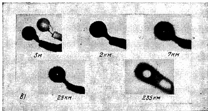
Рис. 275. Фотографии дифракционных картин (тень отбрасывается на экран): а) дифракция от проволоки (I) и карандаша (II); б) дифракция от шурупа; в) дифракция от руки, держащей тарелку, при различных расстояниях от руки до экрана
