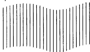
Поперечная волна
