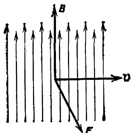
Рис. 349. Направление силы Лоренца F_L , действующей на заряд, движущийся в магнитном поле B со скоростью v . Изображен случай положительного заряда. Для отрицательного заряда сила направлена в противоположную сторону
