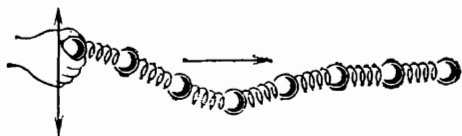
Рис. 71. Поперечная волна
