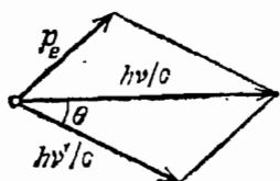
Рис. 372. Упругое столкновение фотона и электрона. До столкновения электрон покоится: h\nu/c — импульс падающего фотона, h\nu'/c — импульс рассеянного фотона, p_e — импульс электрона, \theta — угол рассеяния фотона
