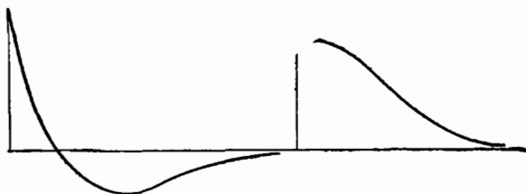
Рис. 23. Апериодические движения
