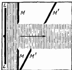
Рис. 170. Волны за широким отверстием распространяются в прямом «канале», проведенном через края отверстия
