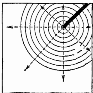
Рис. 78. Кольцевые волны
