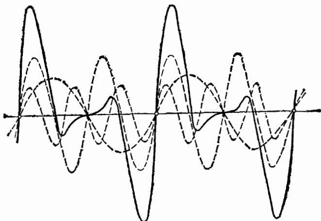
Рис. 33. То же, что на рис. 30, но добавлен второй обертоны
