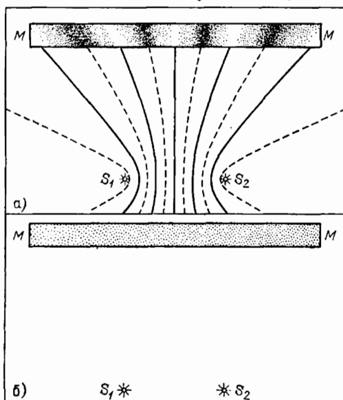
Рис. 93. а) Пластика ММ на пути когерентных волн, пересекающая линии максимумов и минимумов, «освещена» неравномерно. В местах максимумов интенсивность волны больше суммы интенсивностей, в местах минимумов — меньше. б) Если волны некогерентны, то пластинка «освещена» равномерно: интенсивности складываются
