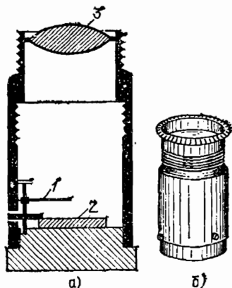
Рис. 382. Спинтарископ в разрезе (а) и внешний вид (б). 1 — иголка, на конце которой находится крупинка радия, 2 — экран из сернистого цинка, 3 — лупа
