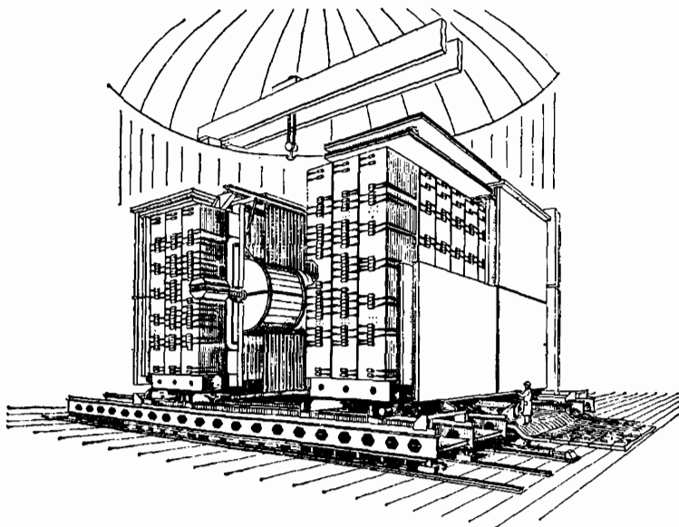
Рис. 422. Общий вид экспериментальной установки UA-1, на которой проводились исследования p\bar{p} -соударений на самом большом в мире ускорителе-накопителе со встречными протонным и антипротонным пучками (SPS-коллайдер ЦЕРН, см. табл. 12). Установка UA-1 — это огромный магнитный спектрометр для измерения импульсов вторичных частиц, образующихся в p\bar{p} -соударениях. Частицы регистрировались в газоразрядной камере (она видна в центре установки). Камера представляет собой совокупность большого числа газоразрядных детекторов частиц, напоминающих пропорциональные счетчики. С помощью этих детекторов определяются траектории частиц. В состав установки входит также большое число сцинтилляционных счетчиков
