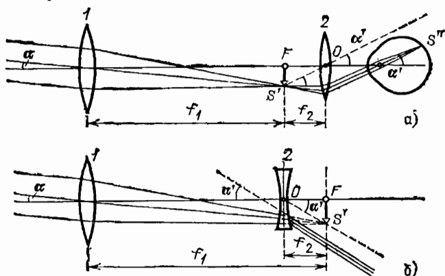
Рис. 254. Ход лучей в зрительной трубе: а) труба Кеплера; б) труба Галлея
