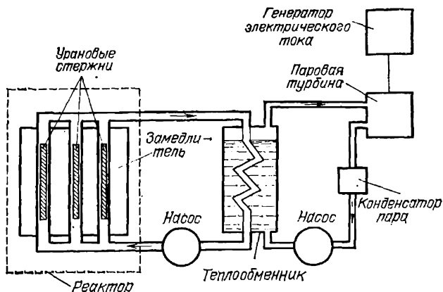
Рис. 409. Принципиальная схема атомной электростанции. Урановые стержни реактора омываются теплоносителем (газом, водой или расплавленным металлом), который отбирает тепло, выделяющееся в стержнях, и в теплообменнике передает его воде, образующей пар. Пар, как и на обычной электростанции, приводит в движение паровую турбину и соединенный с ней электрогенератор. В другом варианте, который также находит применение, пар образуется непосредственно в реакторе, а теплообменник отсутствует
