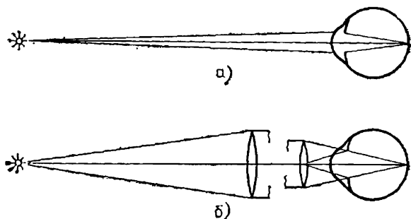
Рис. 260. Световой поток, попадающий в глаз, при использовании телескопа значительно увеличивается
