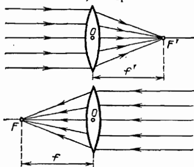
Рис. 196. Фокусы линзы
