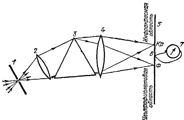
Рис. 297. Схема опыта по исследованию распределения энергии в спектре: 1, 2, 3, 4 — части спектрального аппарата, дающего спектр источника в плоскости 5, 6 — термоэлемент, могущий перемещаться вдоль спектра, 7 — гальванометр, \Phi — фиолетовая граница спектра, Кр — красная граница спектра
