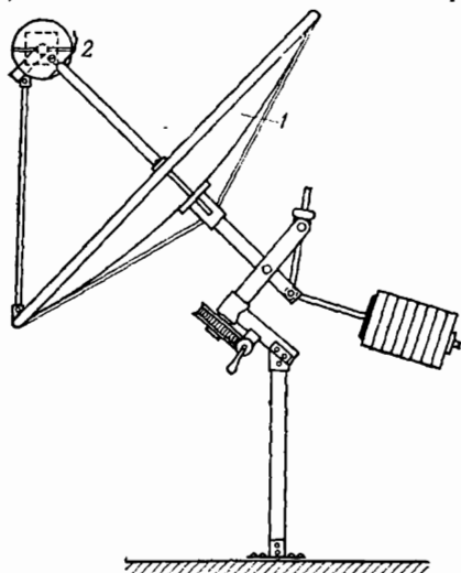
Рис. 152. Схема устройства тепловой солнечной машины: 1 — зеркало, 2 — приемник
