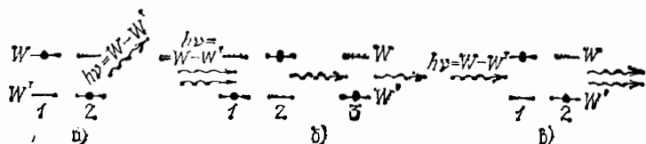
Рис. 361. а) Спонтанное излучение света: 1 — в результате столкновения с другим атомом или с электроном, или в результате поглощения светового кванта атом перешел на один из своих верхних уровней W (для простоты на схеме указаны только два квантовых уровня W и W' ), 2 — через некоторое время возбужденный атом сам по себе (без внешних воздействий) переходит на нижний уровень W' , испуская световой квант h\nu = W - W' . б) Резонансное поглощение света. 1 — атом, находящийся на уровне W' , облучается светом с частотой \nu = \frac{W - W'}{h} (резонансная частота), 2 — атом поглощает из светового пучка один квант h\nu = W - W' и переходит на уровень W ; световой пучок ослабляется; 3 — возбужденный атом при столкновении с другим атомом отдает ему энергию и возвращается на уровень W' (он может вернуться на уровень W' или перейти на другой уровень, расположенный ниже уровня W , также и путем излучения светового кванта). в) Вынужденное излучение света: 1 — атом, находящийся на верхнем уровне W , облучается светом резонансной частоты, 2 — атом испускает квант h\nu = W - W' в направлении падающего светового пучка, который в результате этого усиливается; атом переходит при этом на нижний уровень W' .
