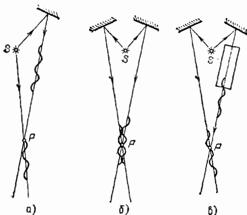
Рис. 264. К интерференции двух пугов световых волн: а) разность хода обоих пугов волн больше длины когерентности — интерференции нет; б) разность хода равна нулю — интерференция есть; в) на пути одного из пугов помещена стеклянная пластинка ( n > 1 ), разность хода обоих пугов больше длины когерентности — интерференции нет
