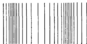
Продольная волна
