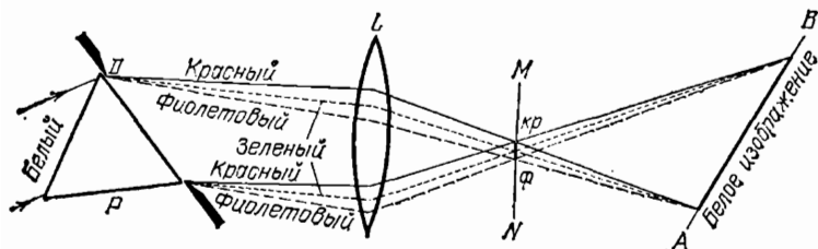
Рис. 312. Схематическое изображение опыта по смещению цветов. Рисунок имеет цветной дубликат (см. форзац)
