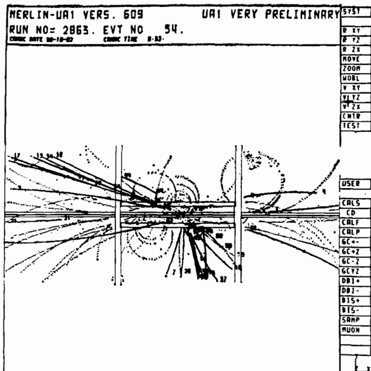
Рис. 423. Снимок с дисплея ЭВМ, работающей вместе с установкой UA-1 (рис. 422). На снимке зарегистрировано одно из p\bar{p} -соударений при энергии 270 ГэВ ( \bar{p} ) + 270 ГэВ ( p ). Информация со всех детекторов установки, обработанная на ЭВМ, позволяет определить траектории частиц и получить полную картину взаимодействия, несколько напоминающую снимки с пузырьковых камер. Импульсы частиц измерялись по кривизне их треков в магнитном поле. Как видно из снимка, взаимодействия при таких высоких энергиях носят очень сложный характер: в них образуется большое число вторичных частиц
