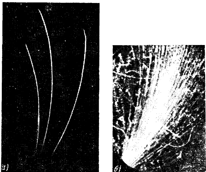
Рис. 380. Следы \alpha - и \beta -частиц в камере Вильсона. Частицы испускаются радиоактивным препаратом, помещенным в нижней части камеры: а) \alpha -частицы: камера в магнитном поле 4,3 Тл, направленном перпендикулярно плоскости рисунка от нас; б) \beta -частицы: магнитное поле 0,0215 Тл направлено на нас
