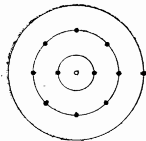
Рис. 369. Схема атома натрия: светлый кружок — ядро атома, черные точки — электроны. Заполнены все места на K - и L -оболочках и один электрон находится на третьей оболочке
