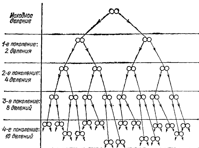
Рис. 404. Развитие цепной реакции деления: условно принято, что при делении ядра испускаются два нейтрона и потеря нейтронов нет, т. е. каждый нейтрон вызывает новое деление; кружочки — осколки деления, стрелки — нейтроны деления
