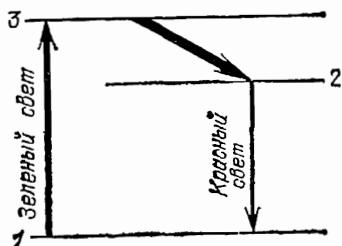
Рис. 363. Схема энергетических уровней атома хрома в рубине
