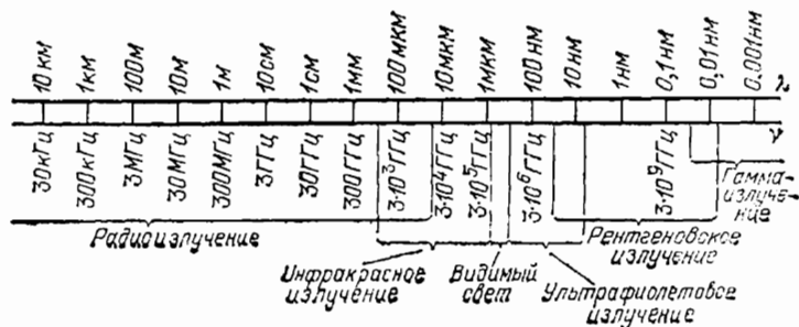
Рис. 125. Шкала электромагнитных волн: 1 ГГц = 10^3 МГц = 10^6 Гц, 1 нм = 10^{-3} мкм = 10^{-9} м
