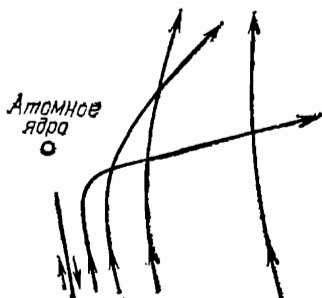
Рис. 358. Траектории \alpha -частиц, пролетающих на разных расстояниях от атомного ядра
