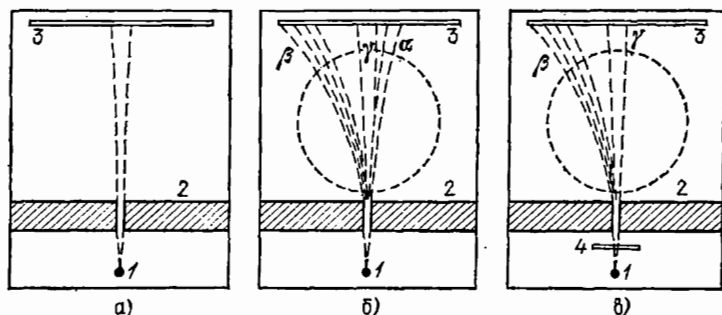
Рис. 377. Отклонение радиоактивного излучения магнитным полем: а) траектории лучей в отсутствие магнитного поля; б) траектории лучей в магнитном поле (штриховой круг — проекция полюсов магнита; линии поля направлены из-за плоскости чертежа на нас); в) лист бумаги толщиной 0,1 мм полностью поглощает \alpha -излучение. 1 — радиоактивный препарат, 2 — свинцовый экран, 3 — фотопластинка, 4 — лист бумаги толщины 0,1 мм
