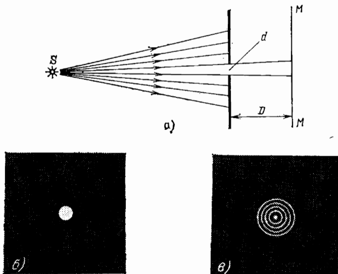
Рис. 274. Дифракция от круглого отверстия: а) схема опыта; б) вид тени, когда диаметр отверстия d сравним с расстоянием D от отверстия до экрана; в) вид тени, когда диаметр отверстия d в тысячи раз меньше расстояния D от отверстия до экрана
