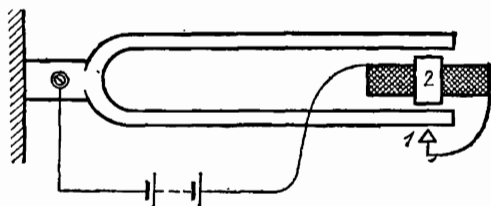
Рис. 56. Автоколебания камертона
