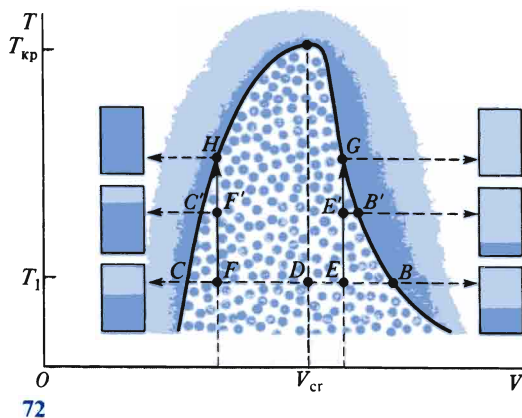
Поведение двухфазной системы при повышении температуры при неизменном давлении
