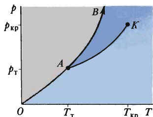
Диаграмма состояний газ – жидкость – твердое тело нормального вещества
