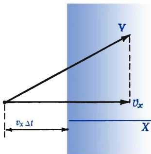
Распределение Максвелла
