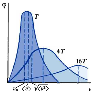
Распределение Максвелла
