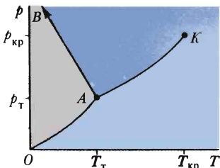
Диаграмма состояний газ – жидкость – твердое тело аномального вещества
