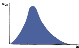
Спектр излучения черного тела
